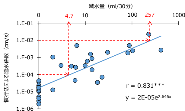
図2 ミニディスクインフィルトメーターによる減水量と慣行法による透水係数との関係
