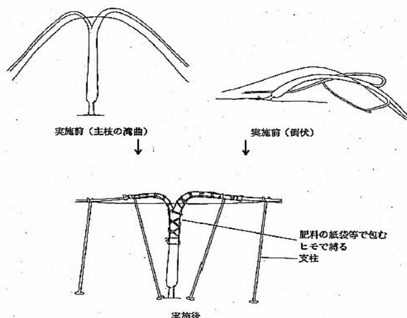
図 1 倒伏樹、主枝の湾曲樹の回復対策 (山梨県)
