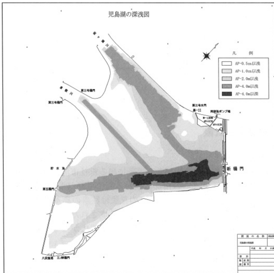
図1-3 児島湖の深淺図（しゅんせつ後）
