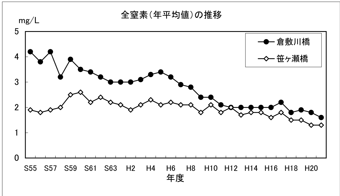
図2-6 流入河川的全窒素(年平均値)の経年変化
