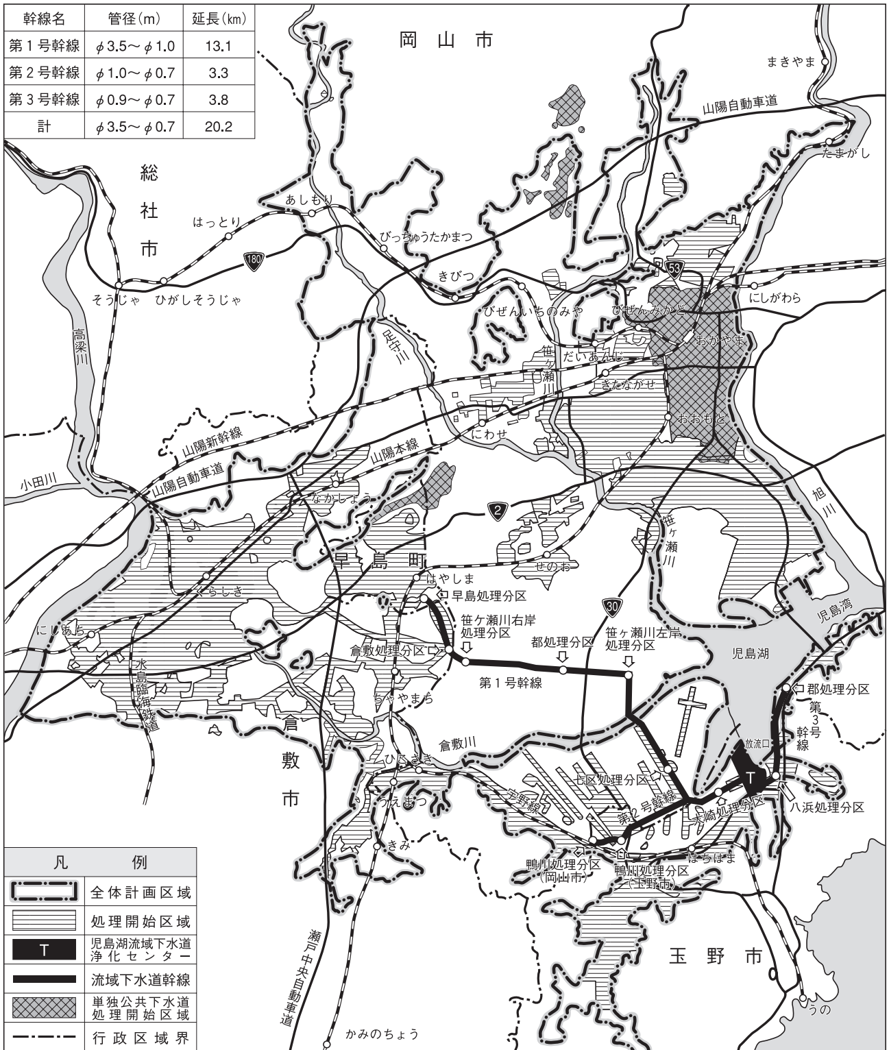
図3-3 児島湖流域下水道事業管内図
