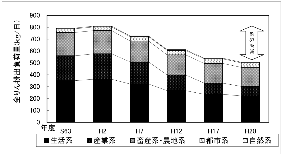
図2-10 全りん排出汚濁量の削減状況
