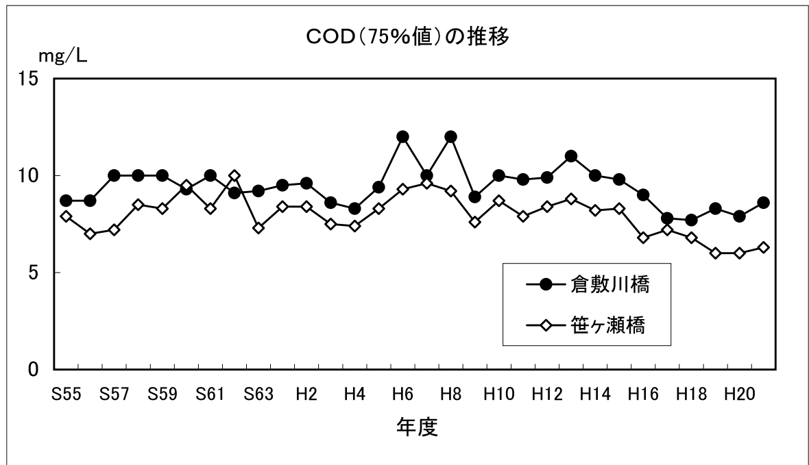
図2-5 流入河川のCOD(75%値)の経年変化
