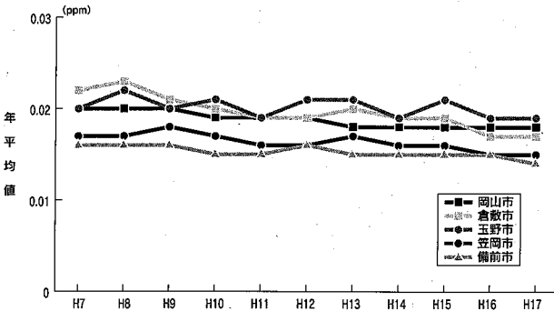
図-2：二酸化窒素濃度の年平均値の推移（一般局）
