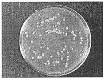
細菌の集落
