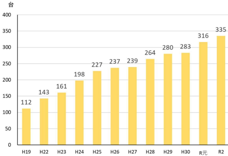
■高性能林業機械の導入状況（岡山県）
