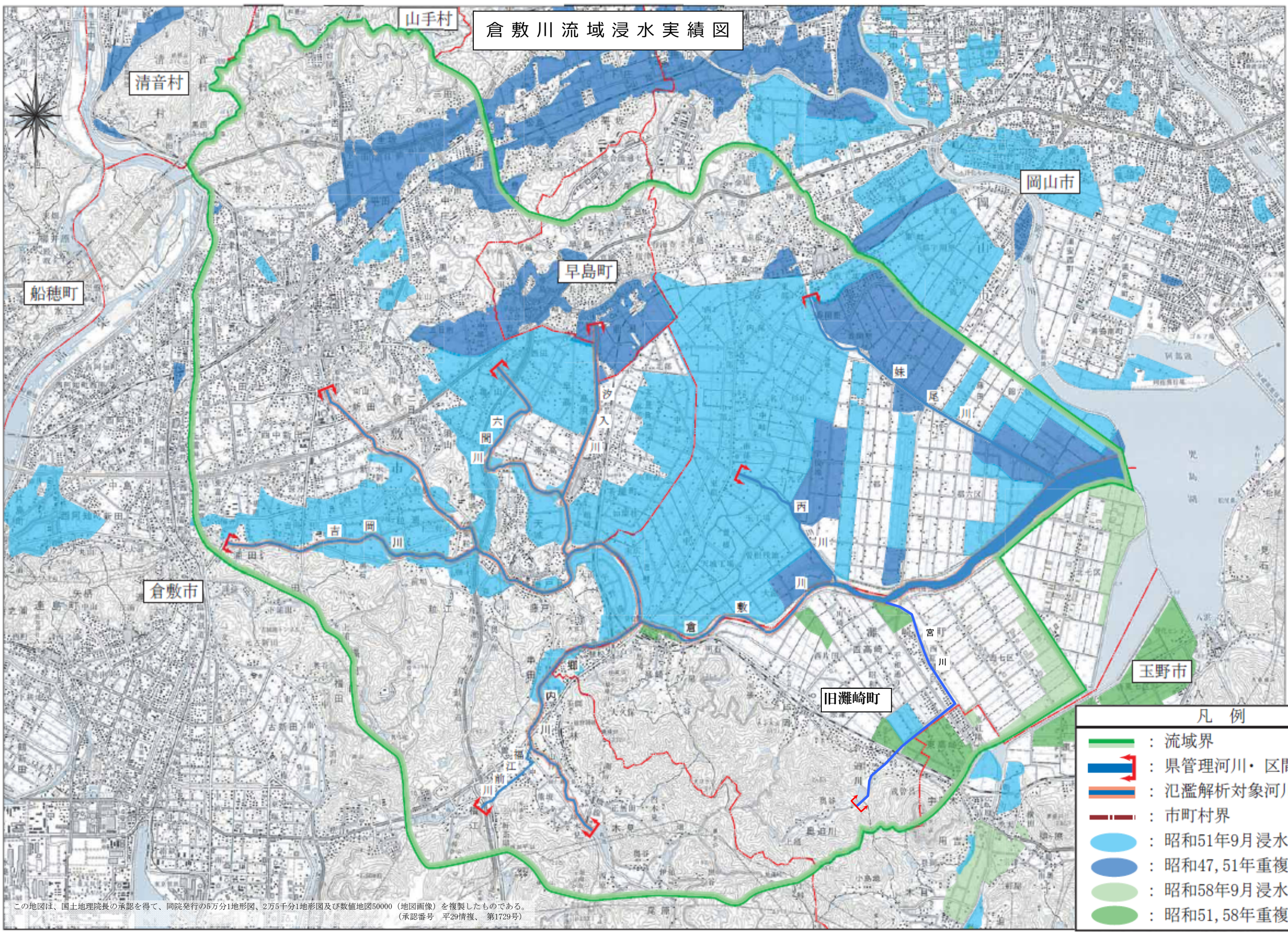
昭和47年7月、昭和51年9月、昭和58年9月の実績浸水区域図（岡山県河川課資料より作成）
