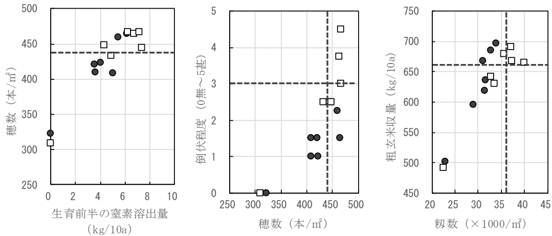
図 1 窒素溶出量と穂数 (左)、穂数と倒伏程度 (中)、籾数と収量 (右) との関係 (2017 年、「中生新千本」) ● 慣行、□ 疎植
