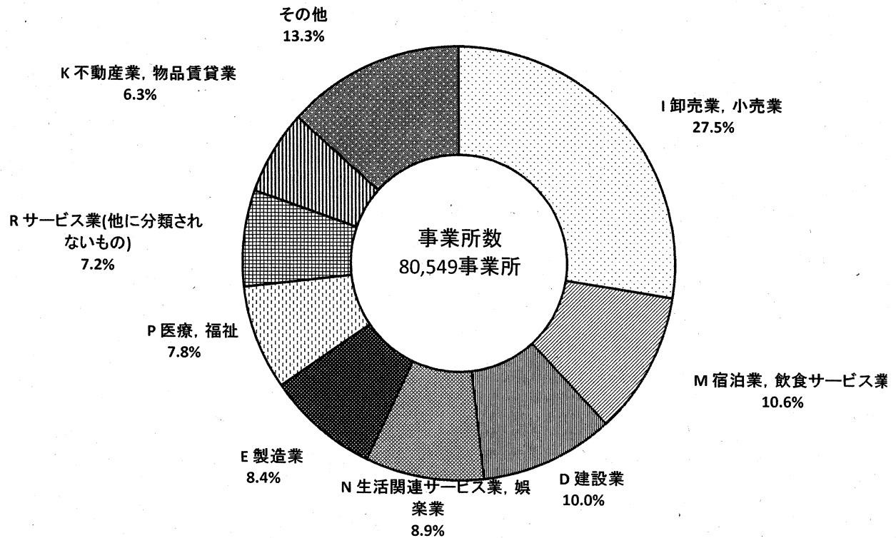
グラフ1 産業別にみた岡山県の事業所割合
