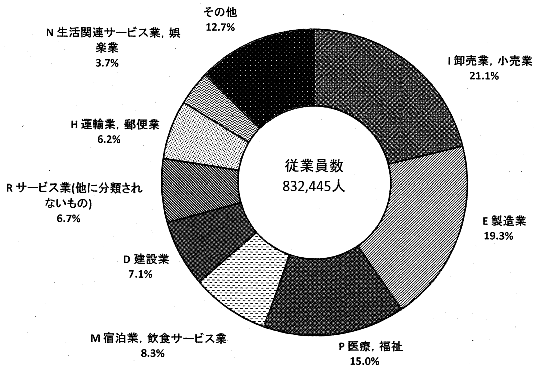
グラフ2 産業別にみた岡山県の従業者数割合
