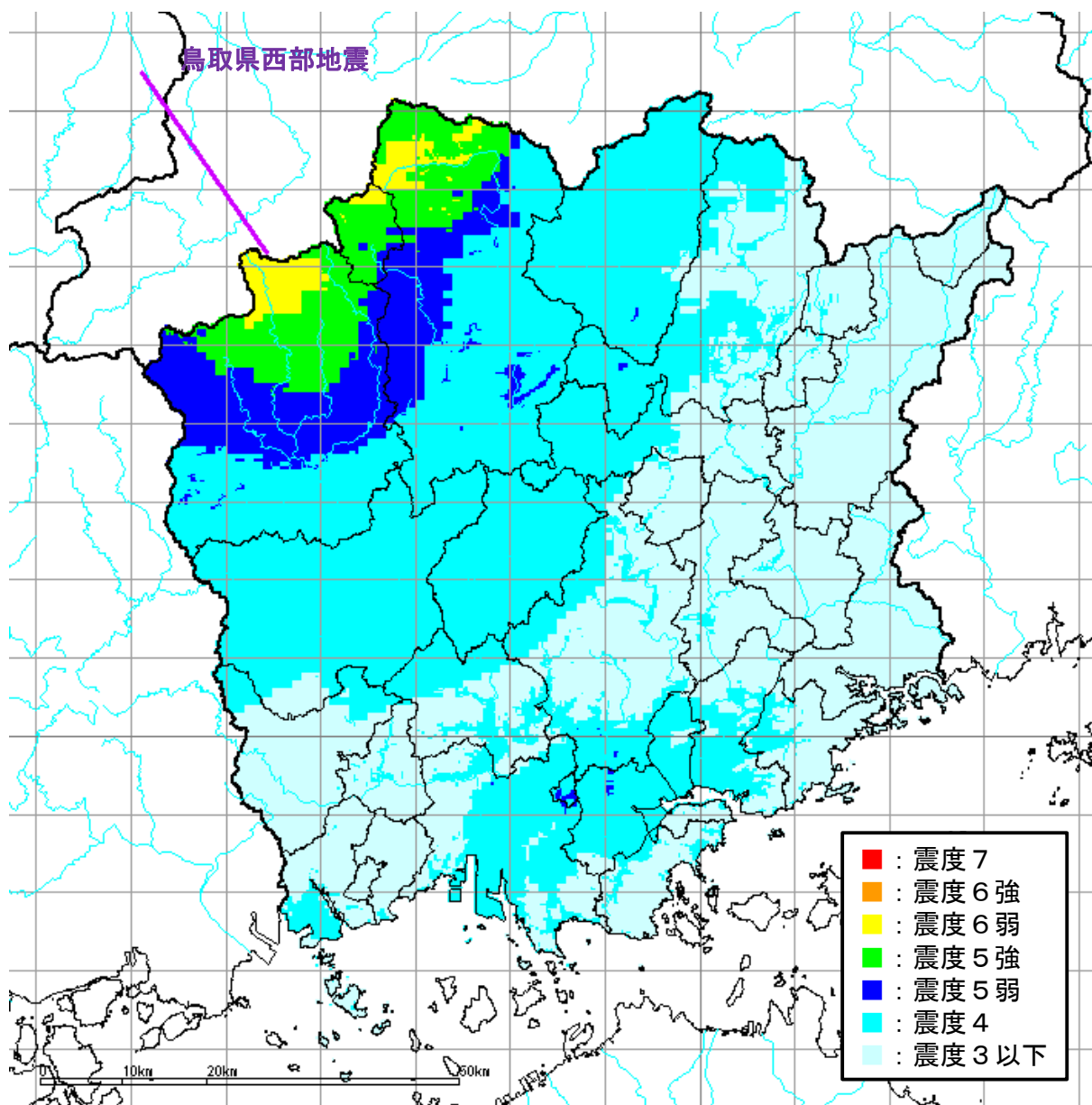
図 9.1.1 震度分布
