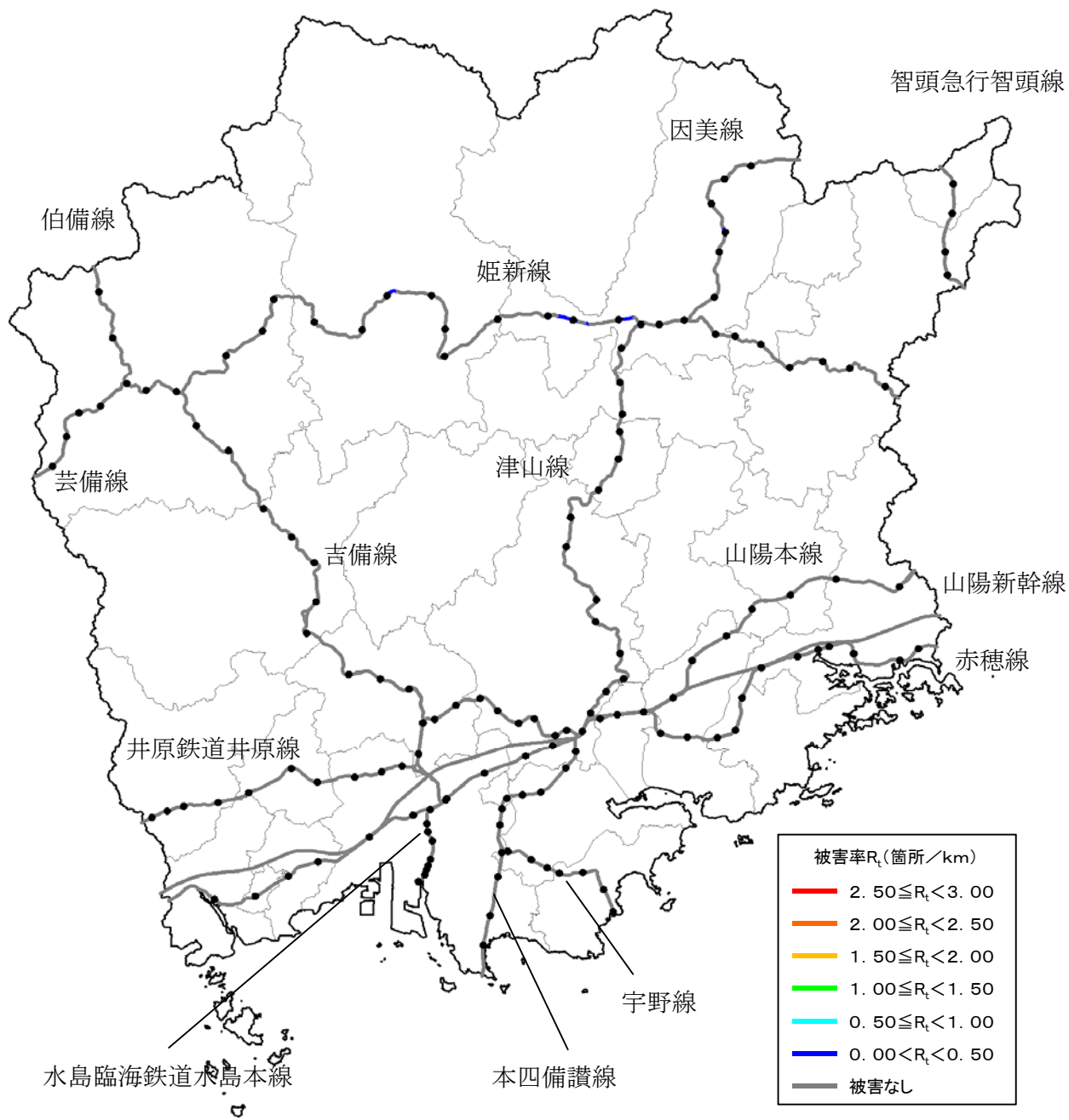
図 7.6.2 鉄道施設被害
