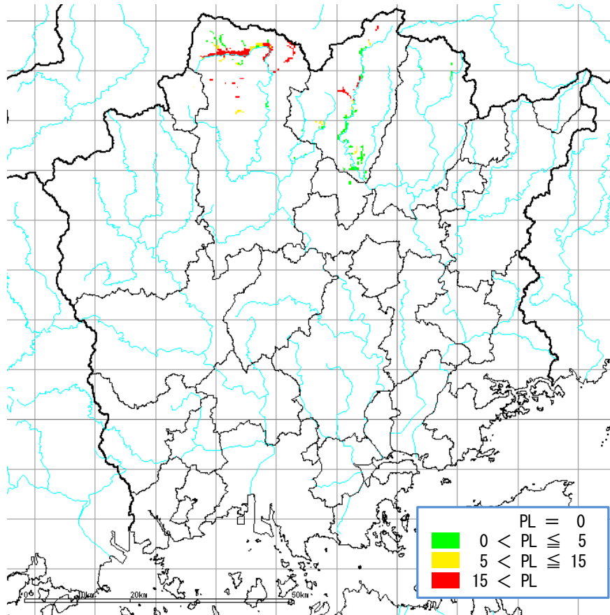
図7.2.1 液状化危険度分布
