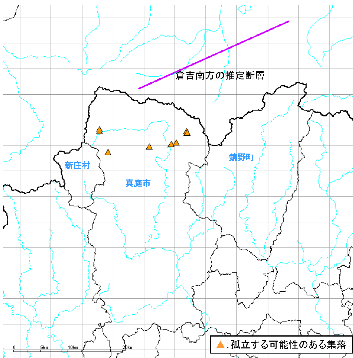
図7.7.1 孤立する可能性のある集落
