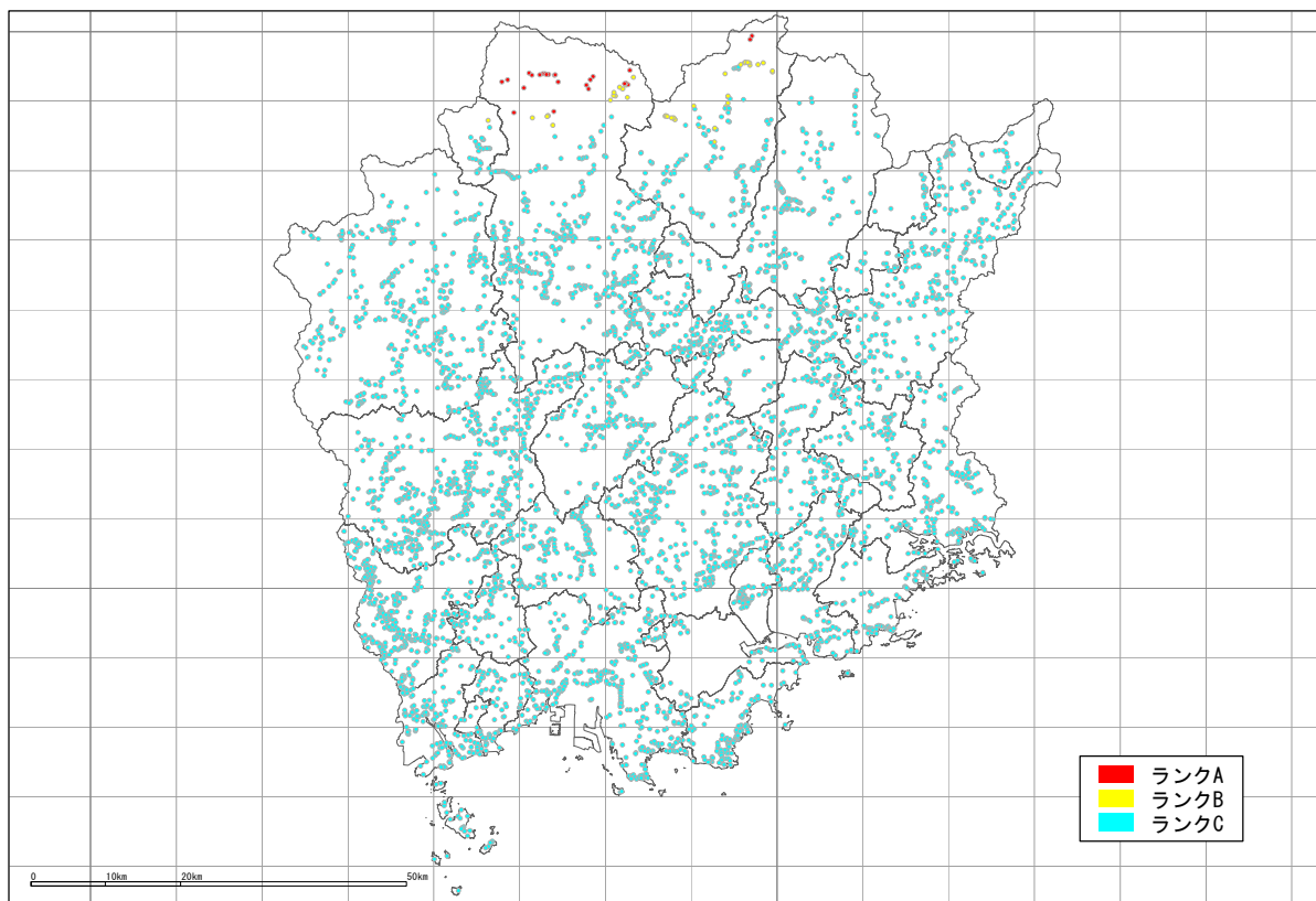
図7.2.2 急傾斜地崩壊危険箇所
