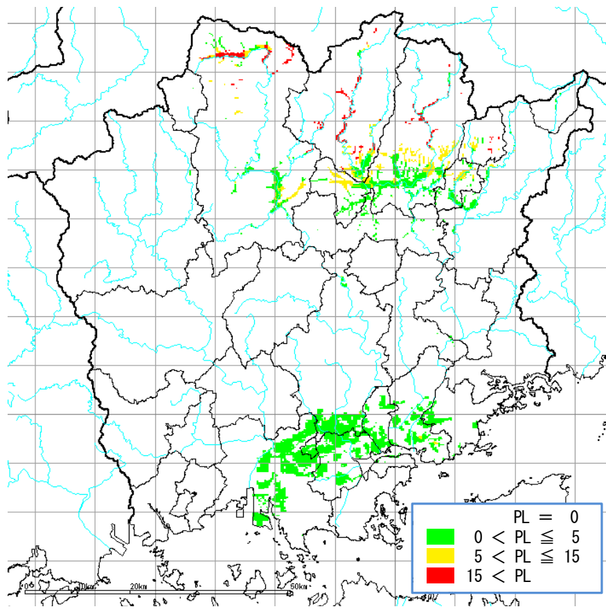
図4.2.1 液状化危険度分布
