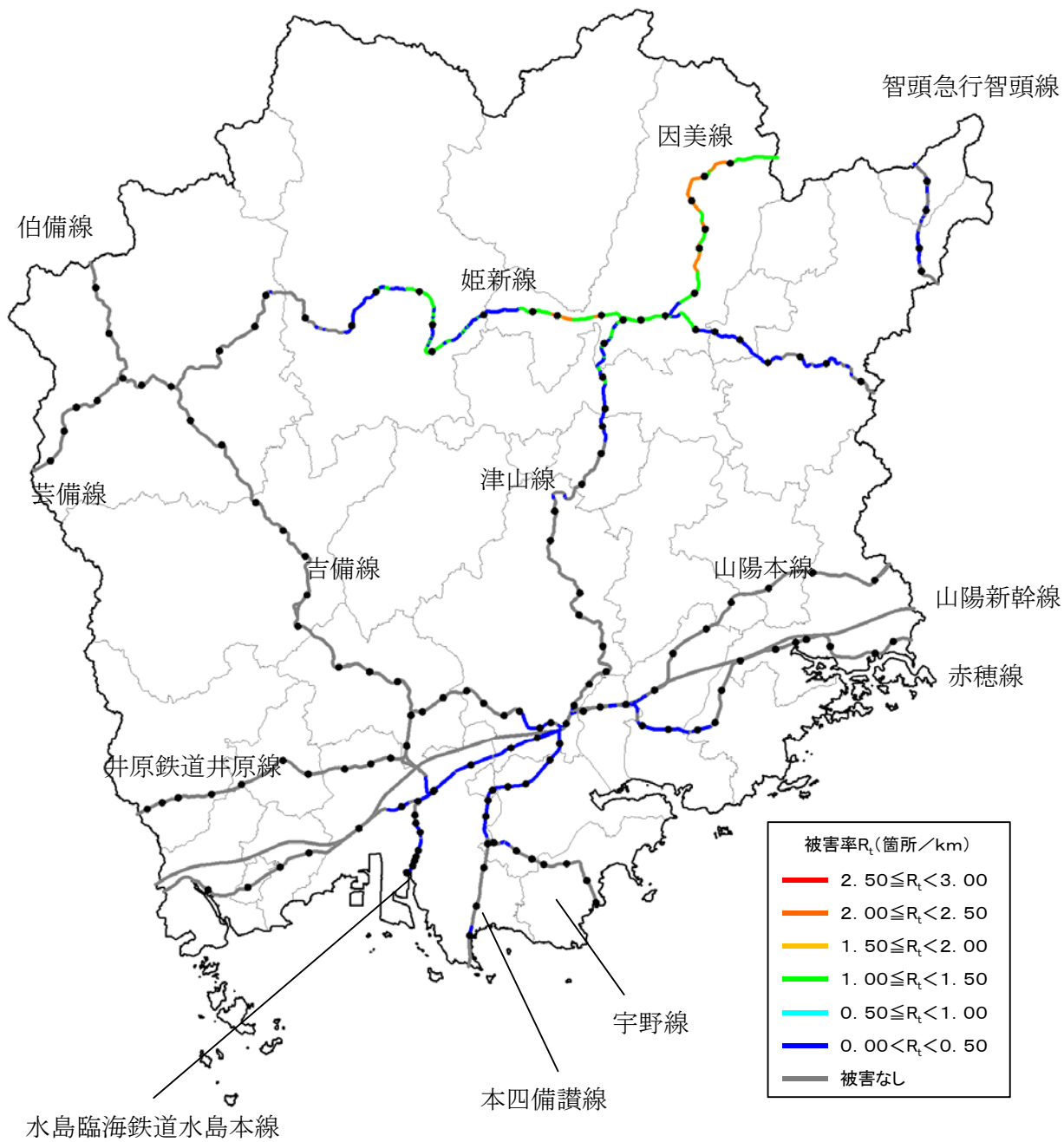
図 4.6.2 鉄道施設被害
