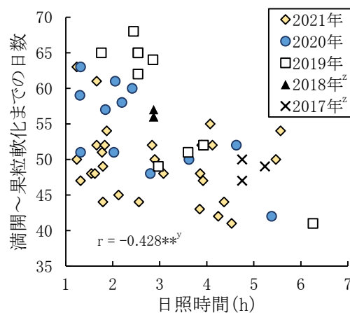
図2 満開日から果粒軟化日までの日数と日照時間 x との関係(n=56)
