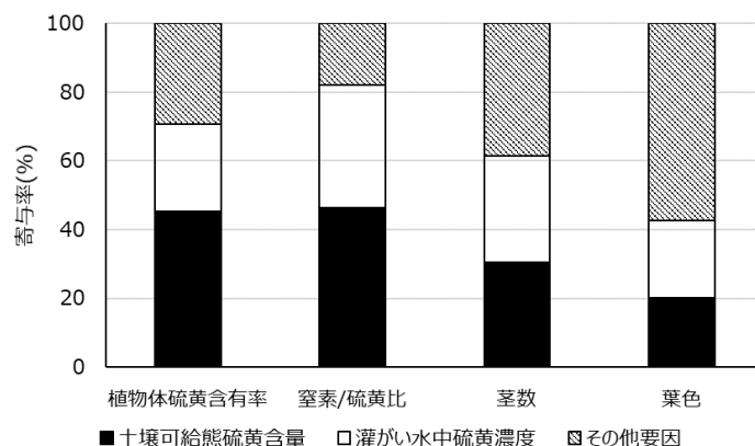
図2 水稻の生育や硫黄診断項目に対する土壌中の可給態硫黄含量と灌がい水中の硫黄濃度の寄与率
