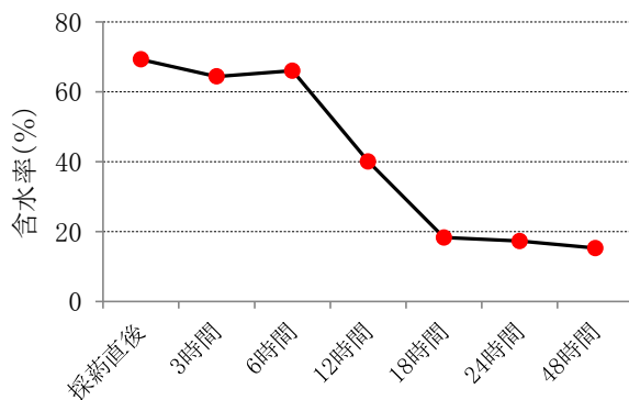
図2 モモ「新白麗」の開薬時間 z の違いが冷凍貯蔵 y 後の粗花粉の含水率に及ぼす影響 z ほぼ25°Cに保った部屋で開薬 y -18°Cで冷凍貯蔵、解凍後の順化なし
