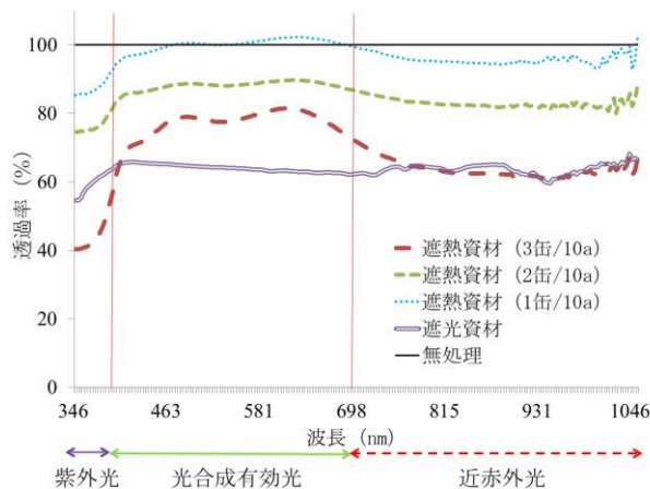
図 1 遮熱資材の処理量及び遮光資材が波長毎の透過率に及ぼす影響 z (2016 年 6 月 21 日 晴天)
