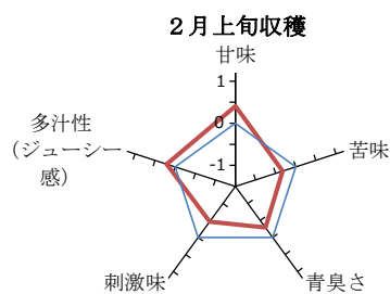
図4 機器分析によって数値化した官能評価値を用いた味のレーダーチャート (それぞれの調査時期の他品種の推定官能評価値を0とした)
