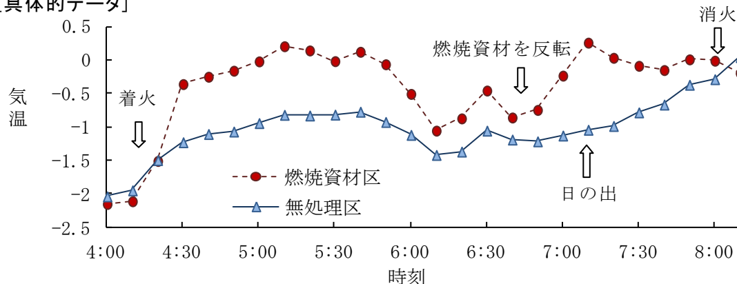
図1 地表から3mの高さの気温 z の推移
