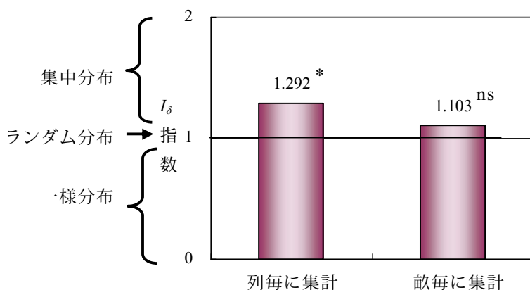
図3 集計方法の違いによる累積発病株の I_d 指数
