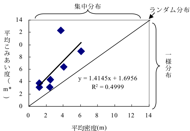
図4 列毎に集計した場合の平均密度(m)と平均こみあい度( m^* )との関係（現地7圃場）
