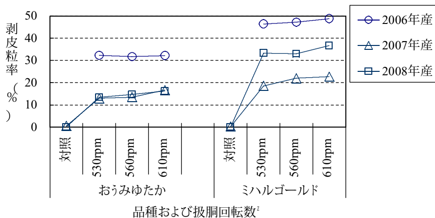
図2 脱穀回転数による剥皮粒の発生状況 1 供試コンバインにおいて、低回転(530rpm、周速度11.1m/s)、適正回転(560rpm、周速度11.7m/s)、高回転(610rpm、周速度12.8m/s)。対照はコンバイン脱穀の影響を受けないように手で脱粒(2006年産はなし)
