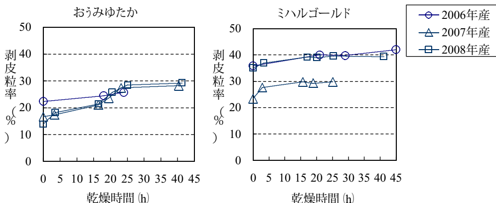
図3 乾燥時間の経過 2 による剥皮粒の発生状況 2 循環型乾燥機 (乾減率: 0.3~0.4%/h) による調査
