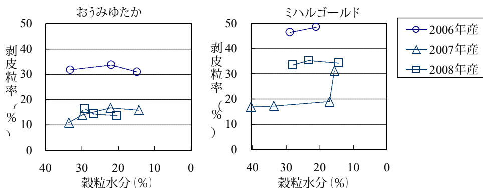
図1 収穫時の穀粒水分による剥皮粒の発生状況
