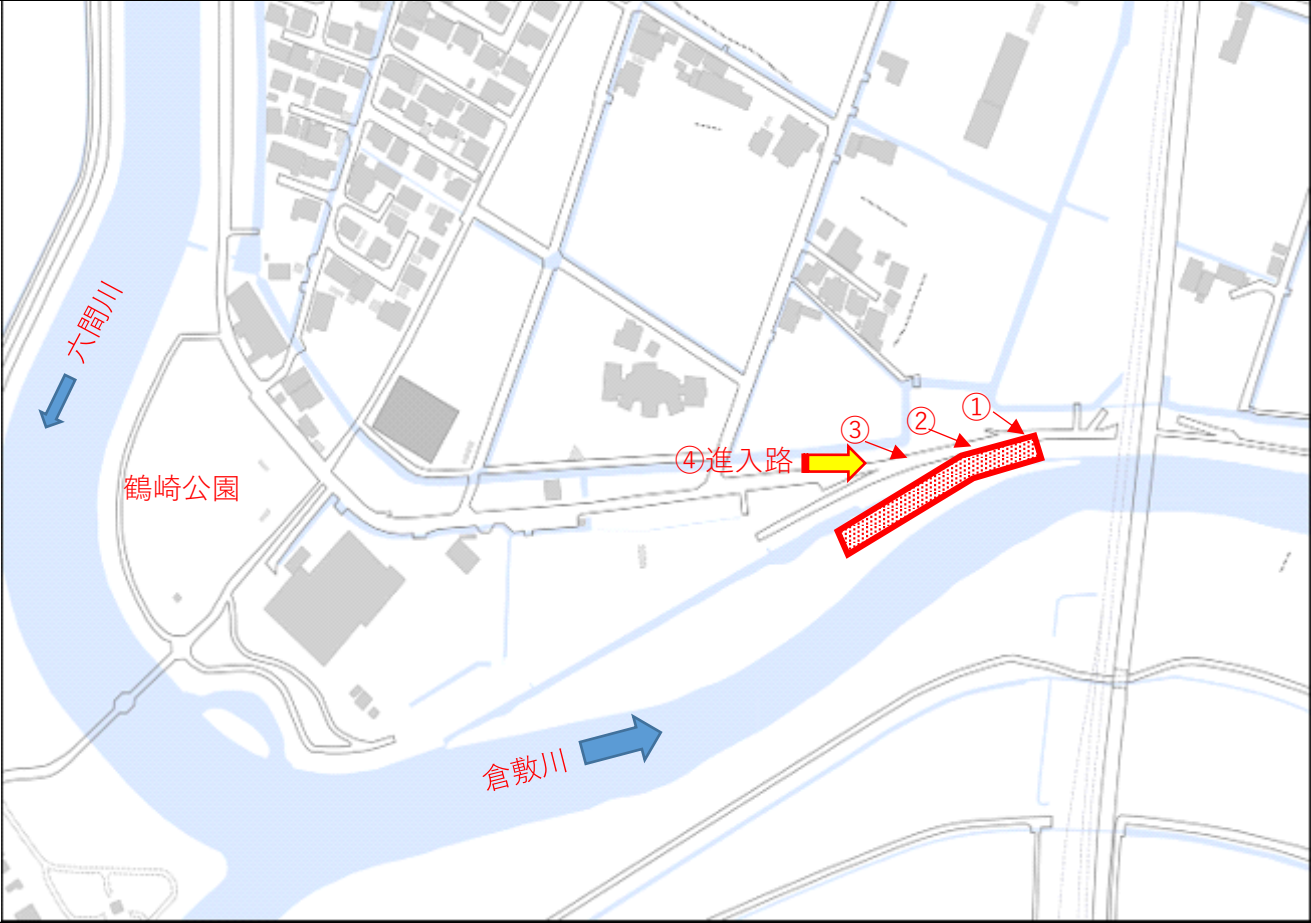
《平面図》
