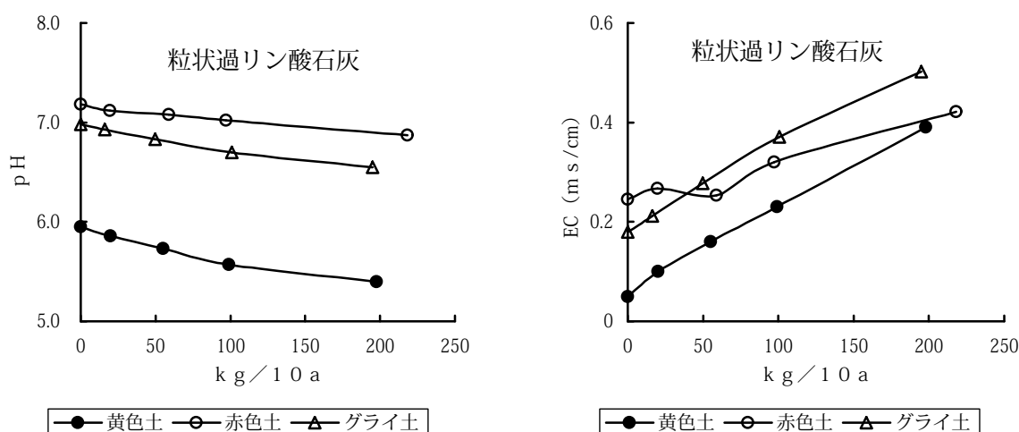
図1 各種土壤に資材を施用した時のpH、EC変化の一例
