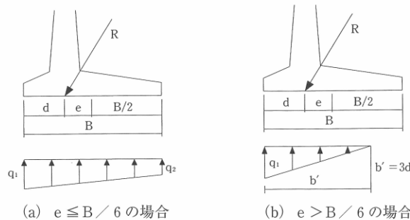
図 3.5.10 擁壁底面の地盤反力分布
