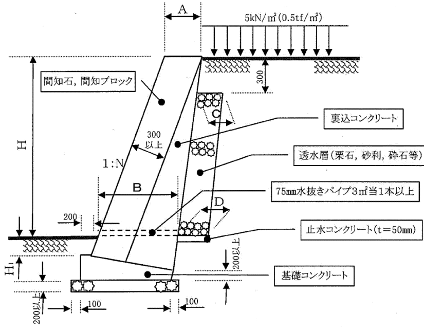
図 3.6.2 練積み造擁壁の標準構造
