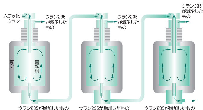
遠心分離機群（カスケード）
