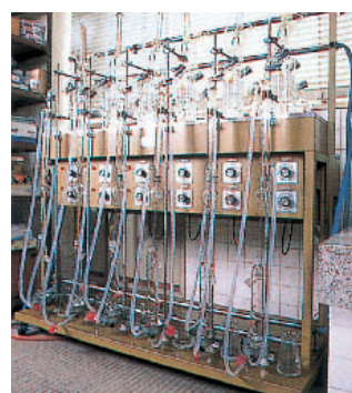
ふっ素蒸留装置
