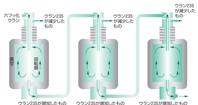
遠心分離機群（カスケード）
