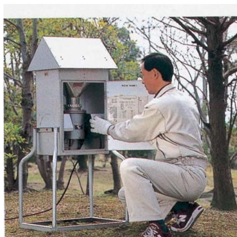
ハイボリューム・エア・サンプラー
