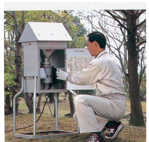
ハイボリューム・エア・サンプラー
