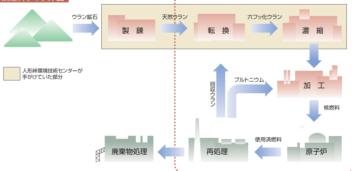
核燃料サイクル図
