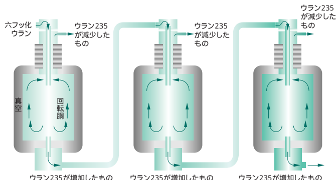
遠心分離機群(カスケード)
