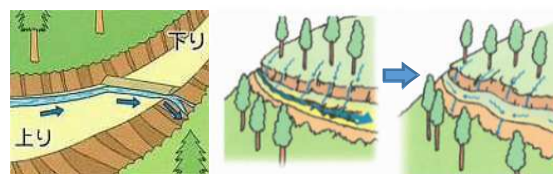
土盛横断排水施設
