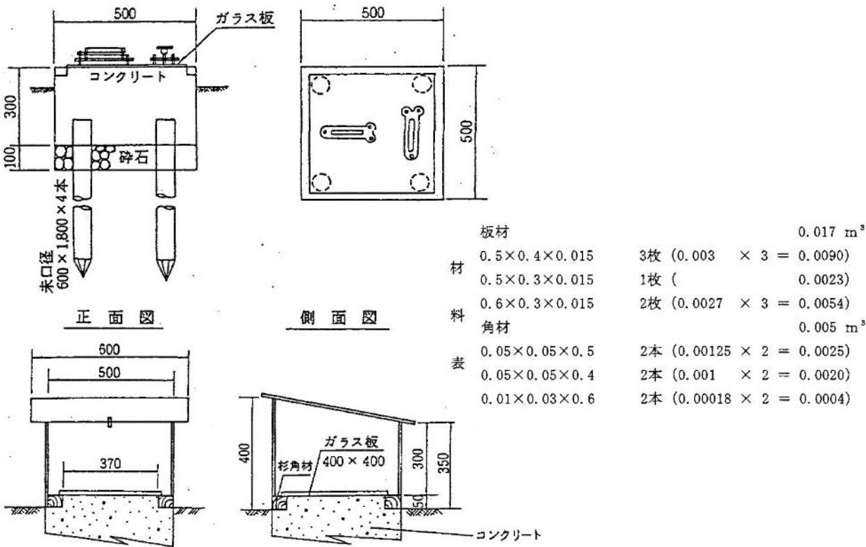
傾斜計構造図（参考図）
