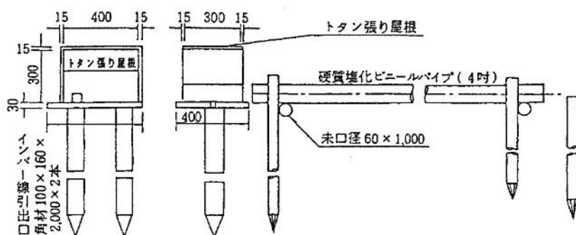
伸縮計構造図 (参考図)
