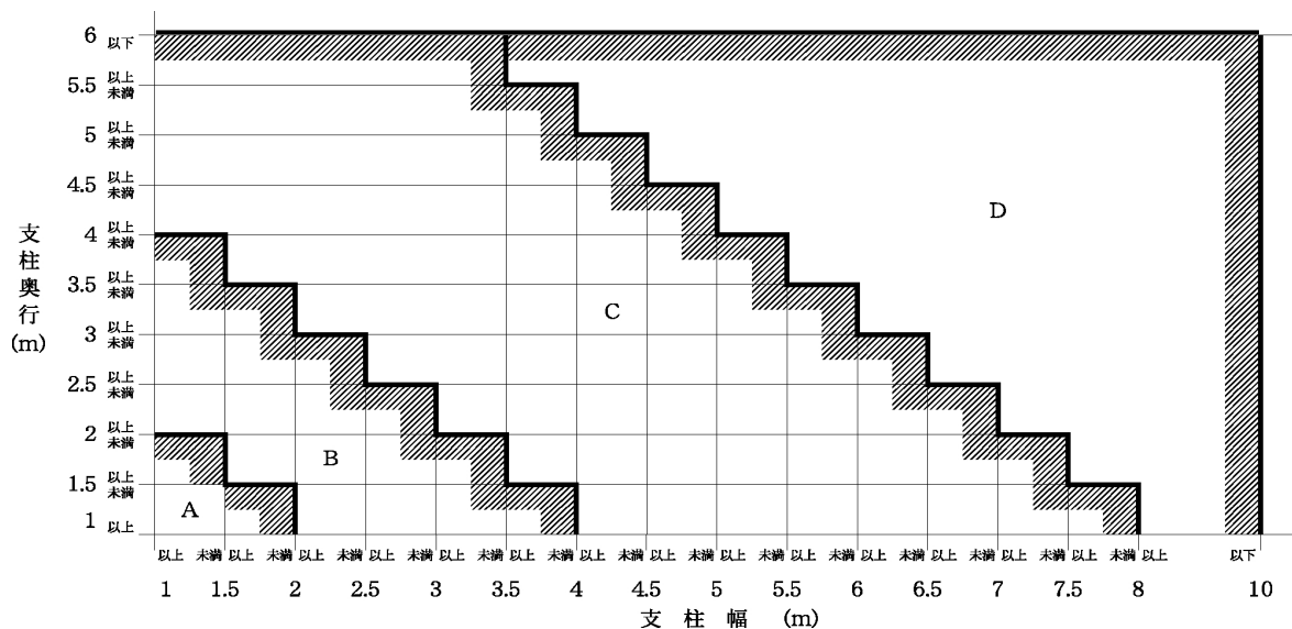
図1-1 矩形(小判形を含む)支柱の適用範囲
