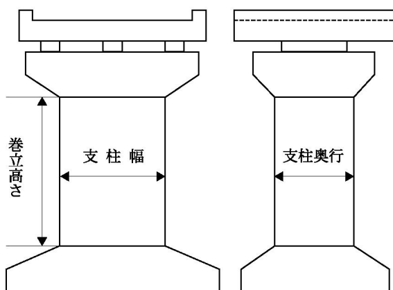
(1) 矩形（小判形を含む）支柱
