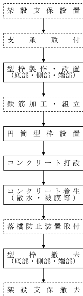
図2-1 施工フロー
