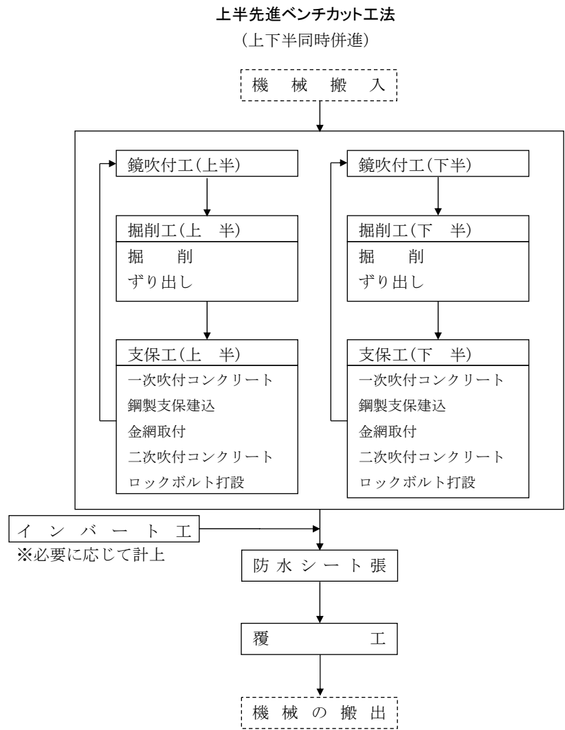
図2-1 施工フロー
