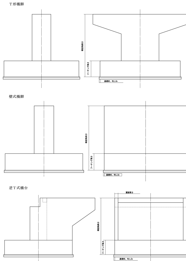
橋台・橋脚形式(参考図)
