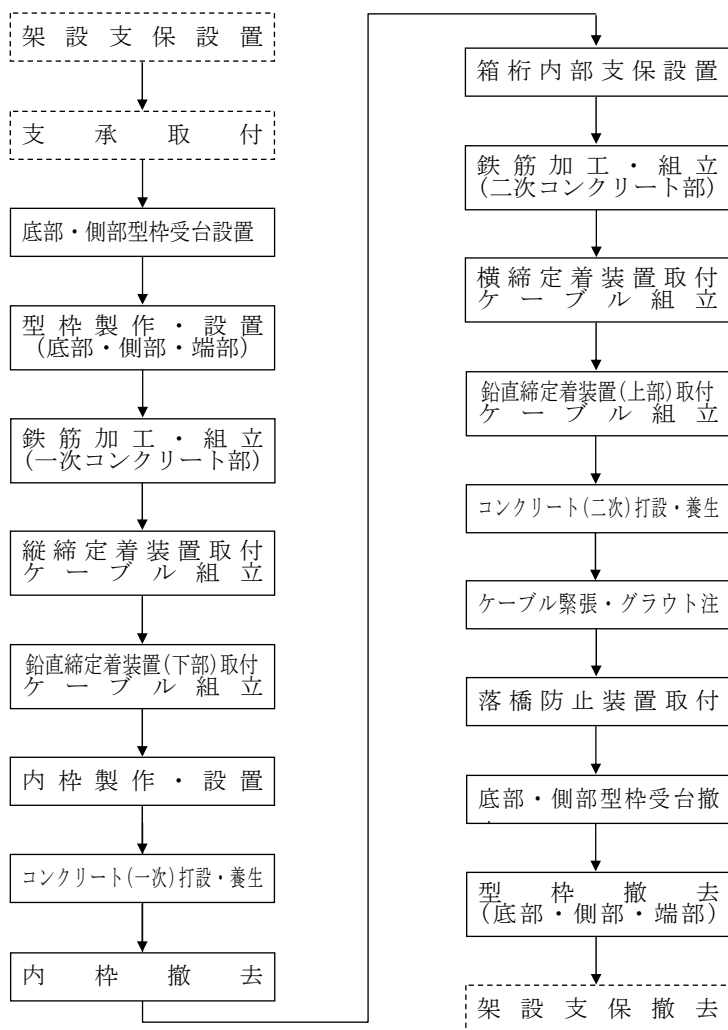
図2-1 施工フロー
