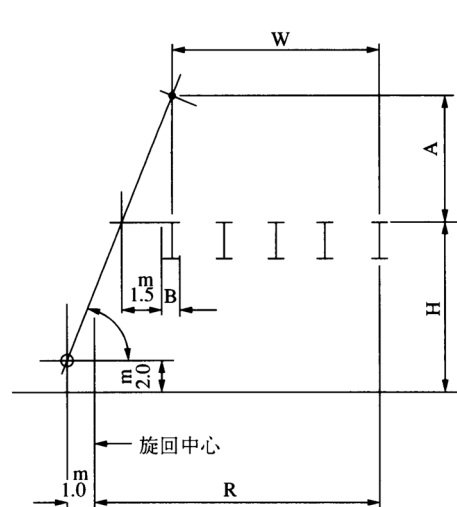
図 17-2 作業半径算定式
