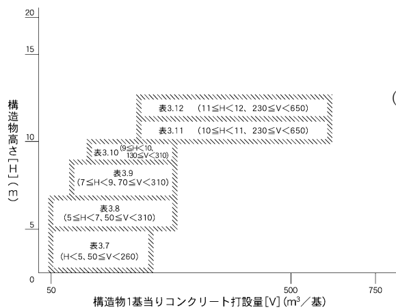
図3-3 逆T式橋台歩掛表適用範囲
