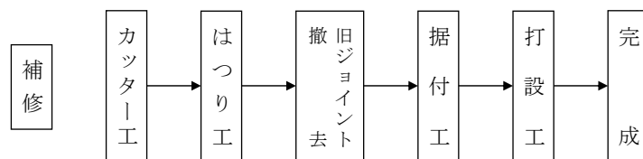
図4-1 施工フロー(鋼フィンガージョイント等から既製品ジョイントへの取替え)
