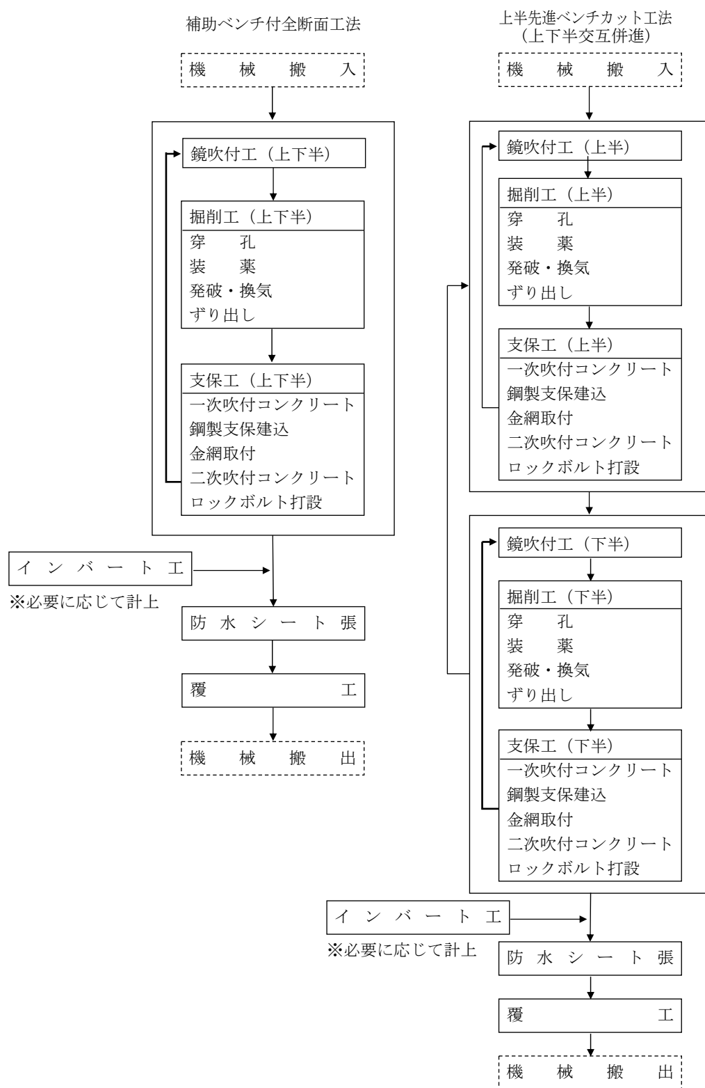
図2-1 施工フロー
