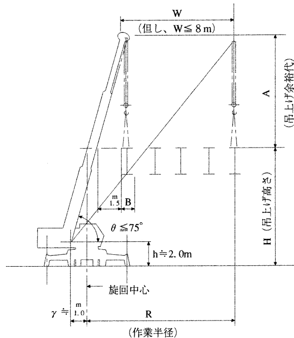
図 17-1 作業半径概略図・鉋桁(移動式クレーン油圧伸縮ジブ型)
