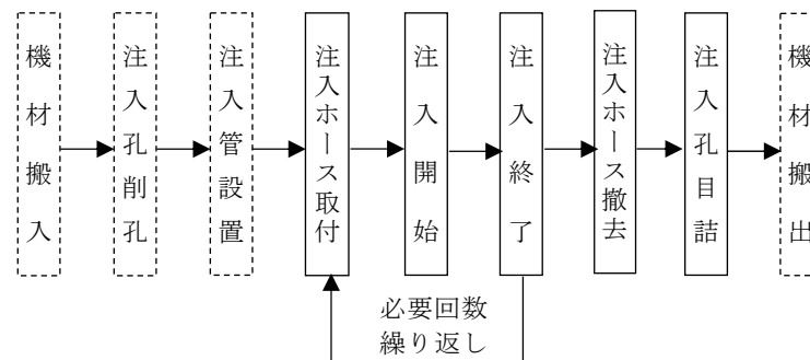
図2-2 施工フロー
