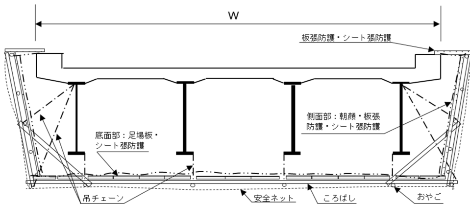
パイプ吊足場参考図
