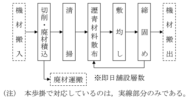
図2-1 施工フロー
