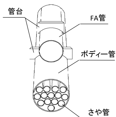
FA 管・ボディー管 (管路材参考図)
