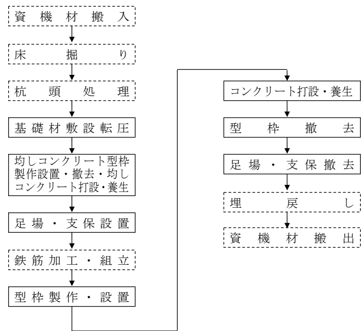
図2-1 施工フロー
