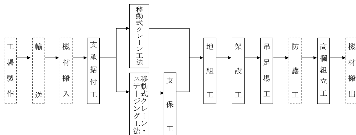
図2-1 施工フロー
