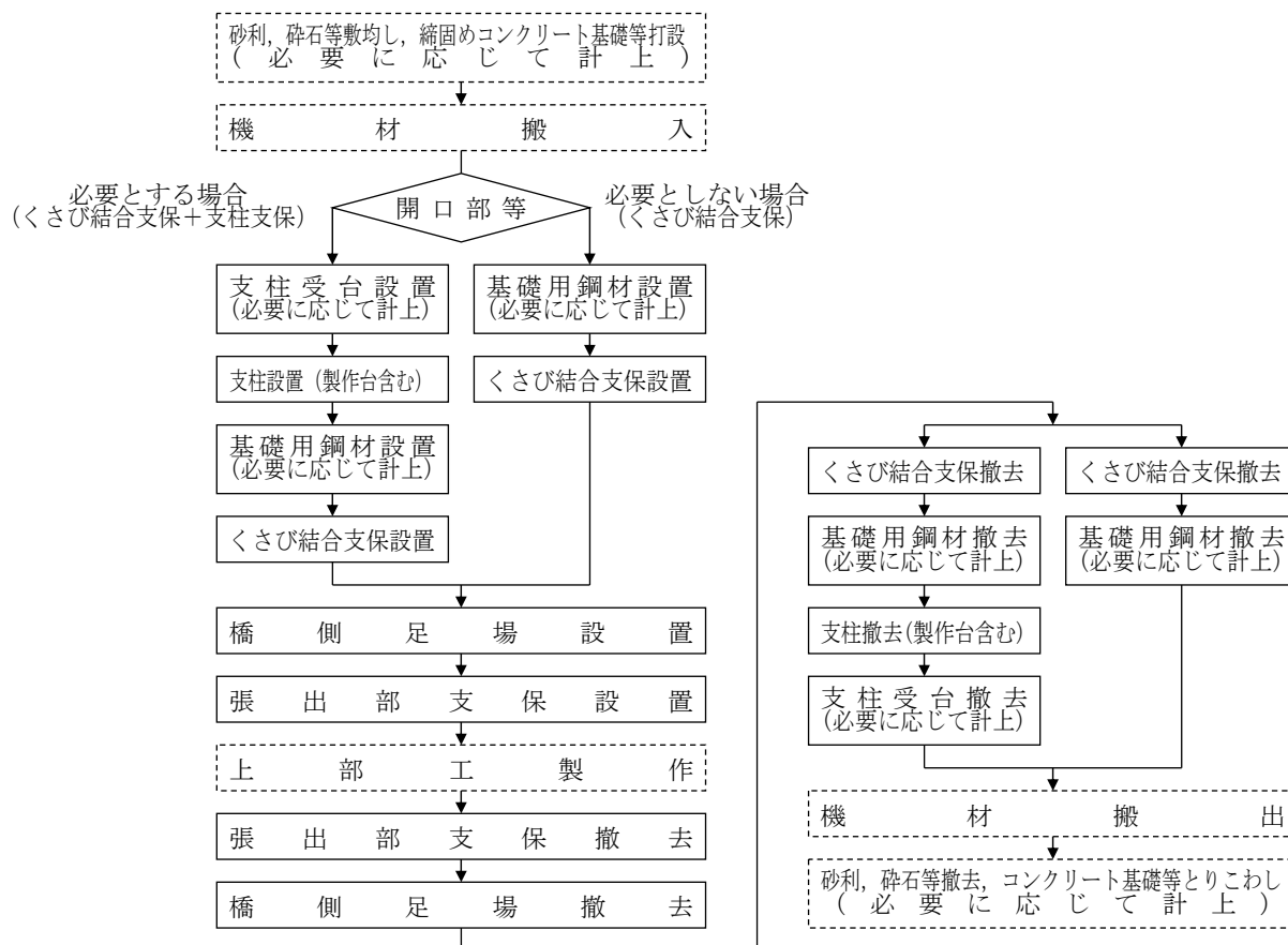
図2-1 施工フロー
