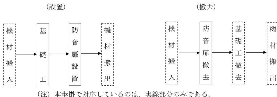
図2-1 施工フロー
