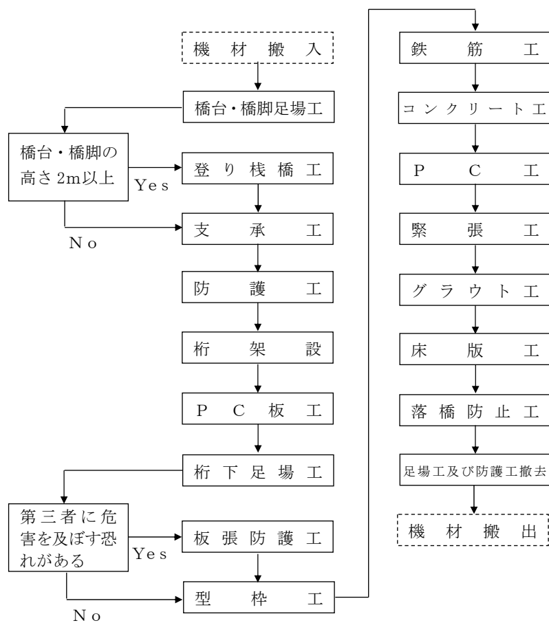
図2-2 施工フロー
