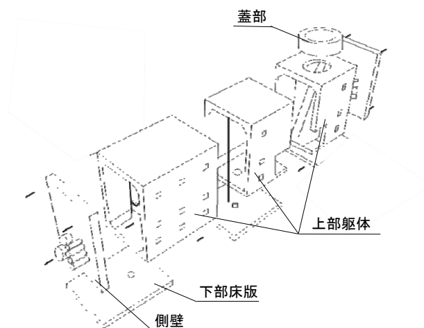
（プレキャストボックスブロック参考図）
