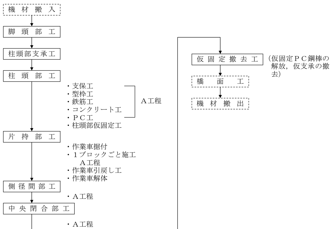
図2-1 施工フロー
