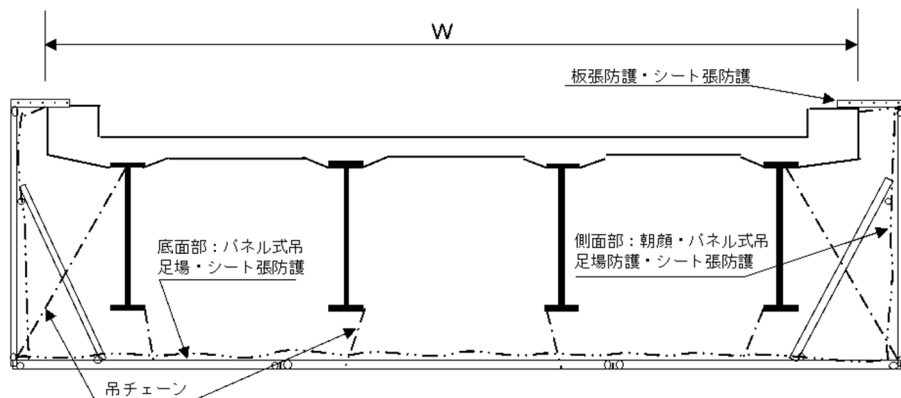
システム(パネル式)吊足場参考図
