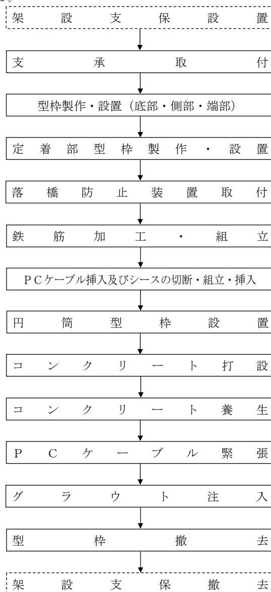
図2-1 施工フロー
