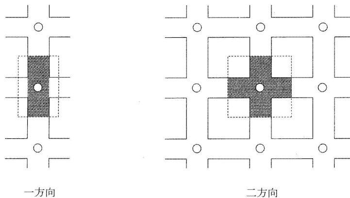
アンカーの荷重分担
