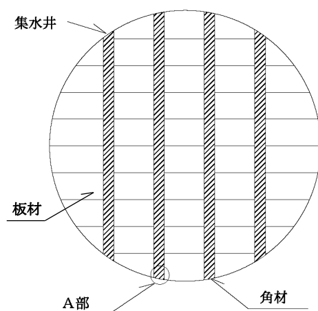
(2) [参考図] 集水井内足場概念図 平 面 図
