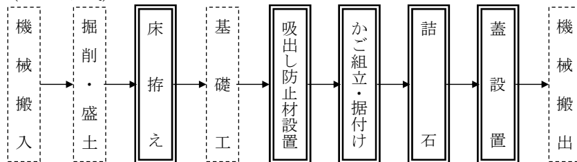
図2-1 施工フロー(じゃかご)
