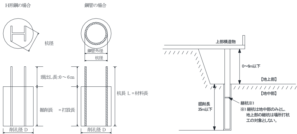
図1-1 施工図
