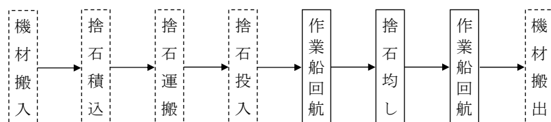
図2-1 施工フロー
