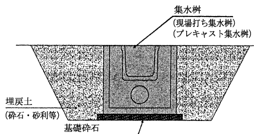
図8-4 集水樹 構造概念図
