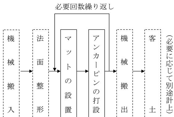
図2-1 施工フロー
