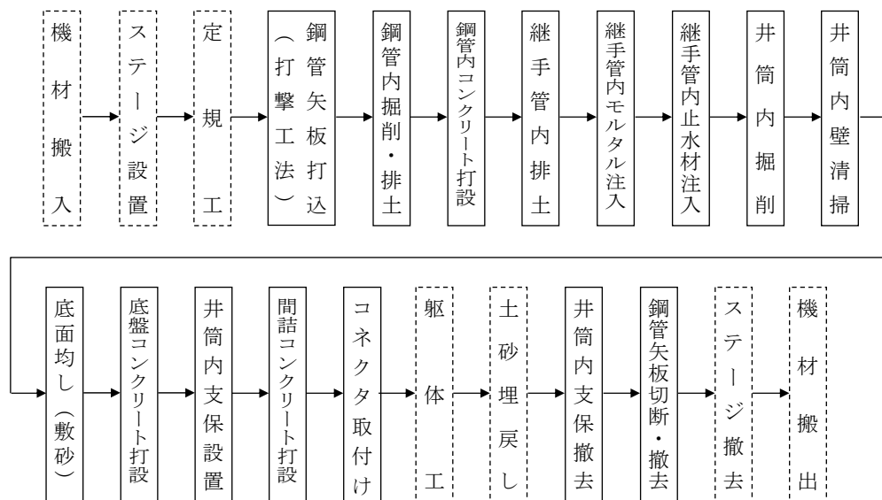
図2－1 施工フロー
