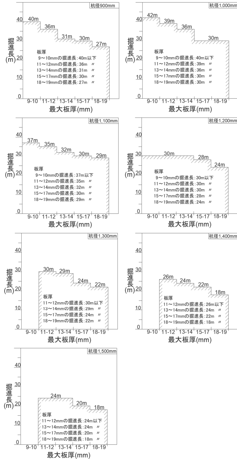
図1-1 適用掘進長
