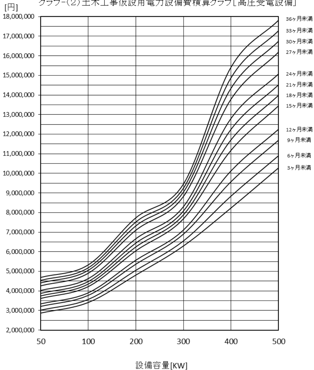
グラフ-(2) 土木工事仮設用電力設備費積算グラフ[高圧受電設備]
