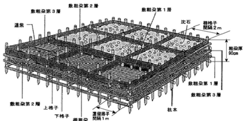
図3-1 参考図(粗朶沈床概念図)
