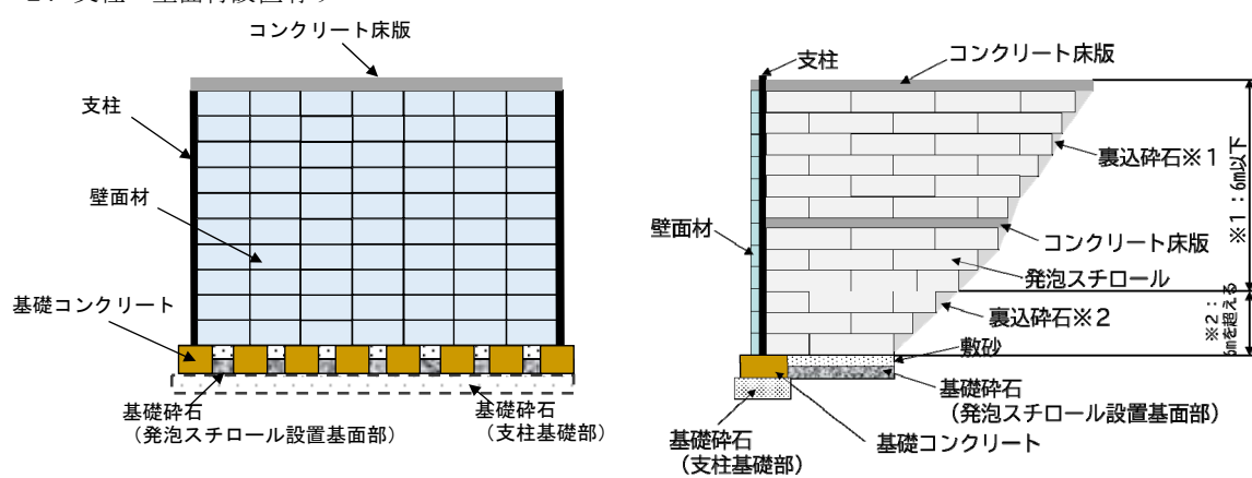
片側壁図
