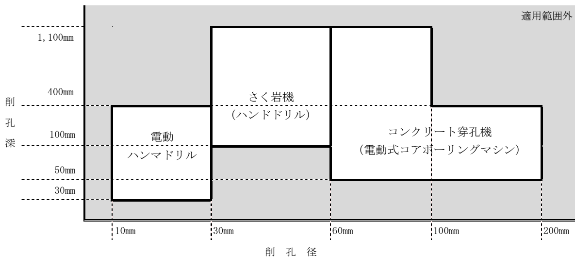
図1-1 削孔機械の選定
