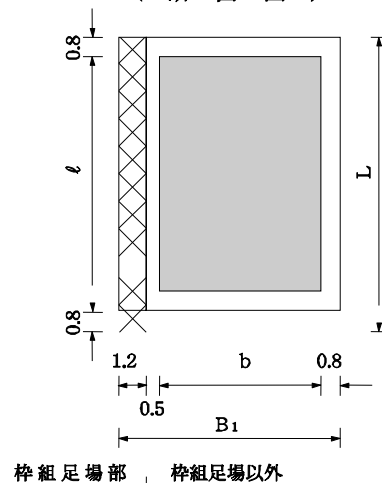
(平面図)
