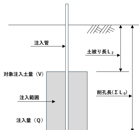
図3. 1 施工図(二重管ストレーナ工法)
