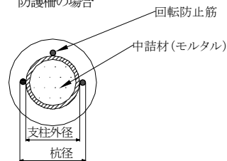
防護柵の場合
