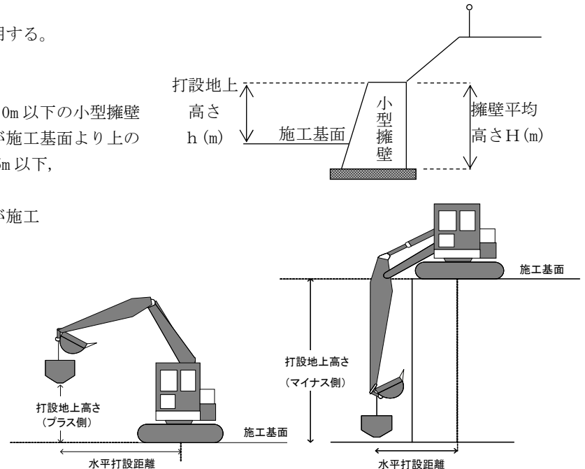
参考図(バックホウによるコンクリート打設範囲)
