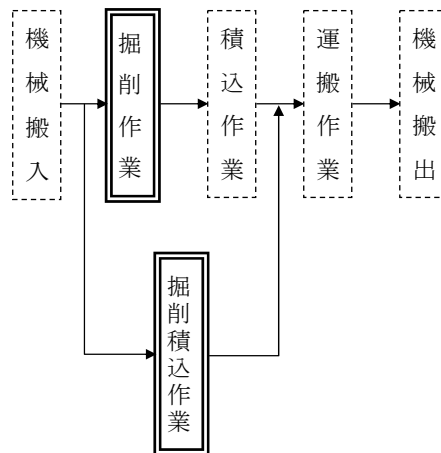
図2－1 施工フロー
