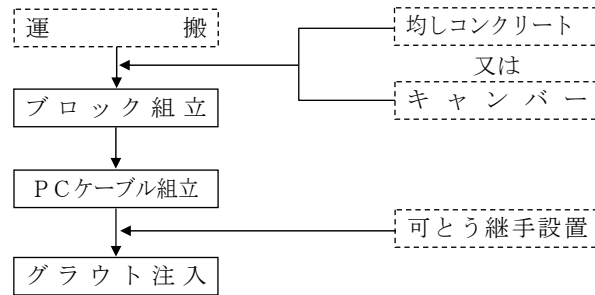
図2-1 施工フロー
