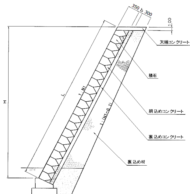
参考図 石積(練石)(複合)の断面図
