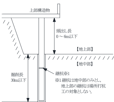
鋼管・H形鋼の場合
