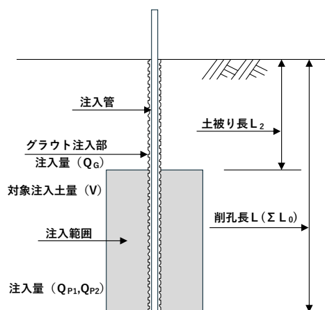
図3. 2 施工図(二重管ダブルパッカー工法)
