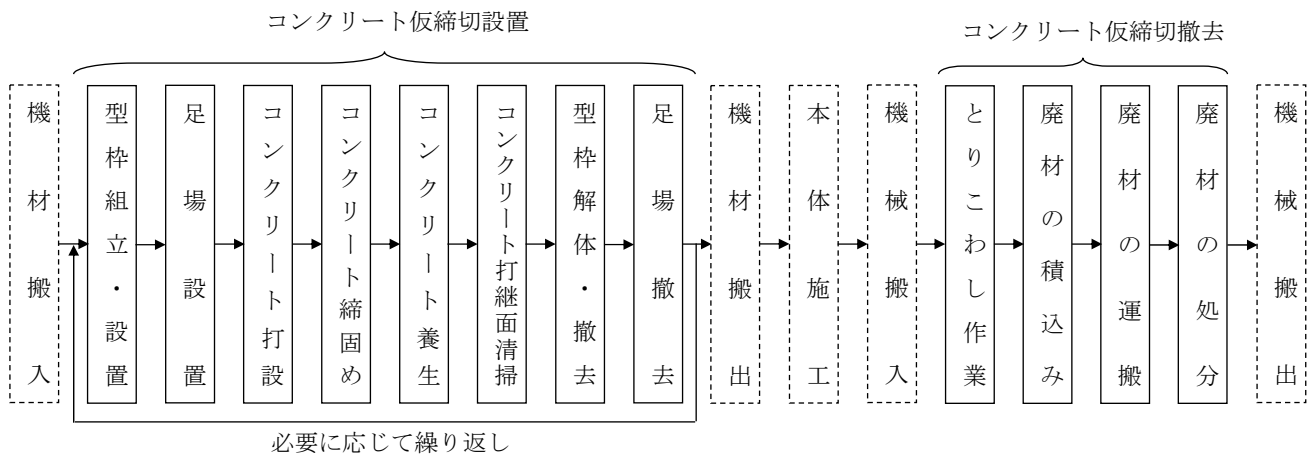
図2－1 施工フロー
