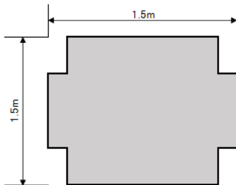
帯鋼補強土壁正面図
