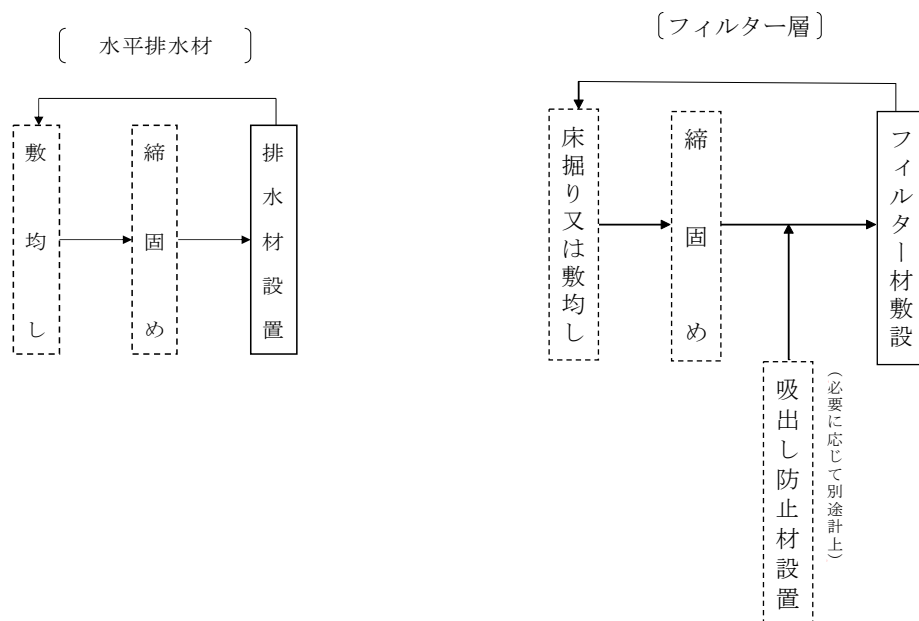
図2-1 施工フロー
