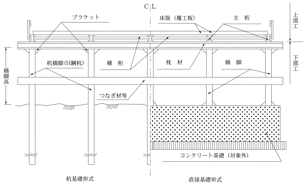
図2-2 仮橋・仮栈橋工概念図
