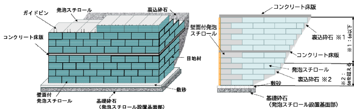
片側壁図
