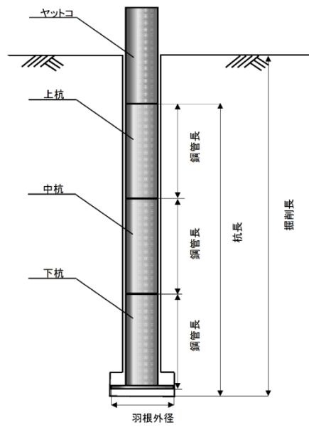
図 1-1 施工図
