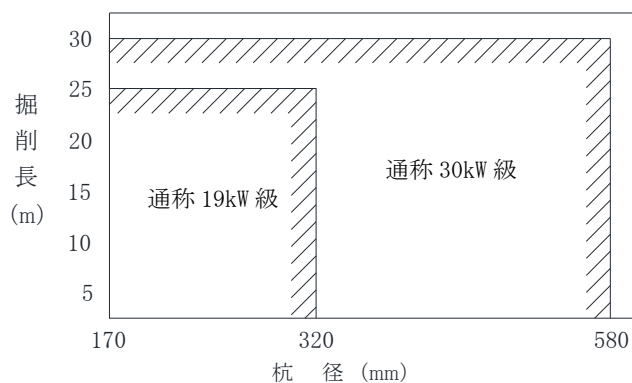
図3-1 大口径ボーリングマシンの選定
