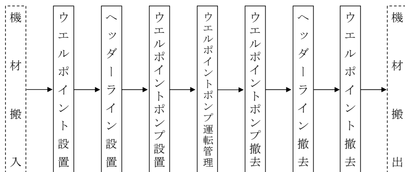
図2-1 施工フロー
