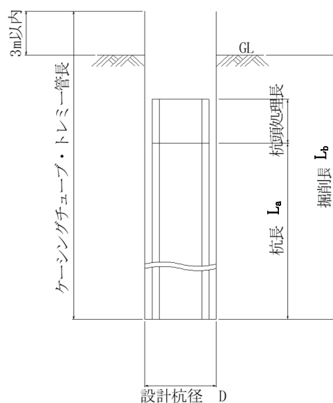
図5-1 施工図
