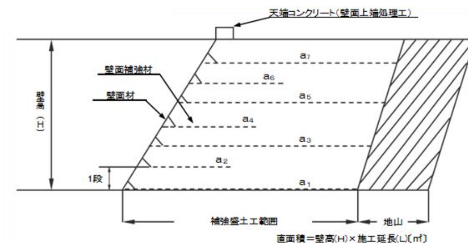
図3-1 補強盛土工標準断面図(参考図)
