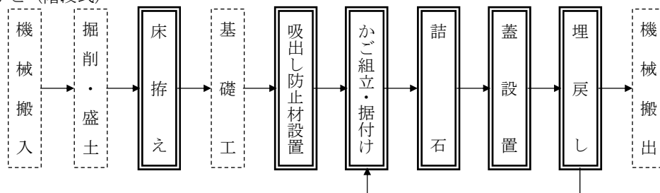
図2-3 施工フロー(ふとんかご(階段式))
