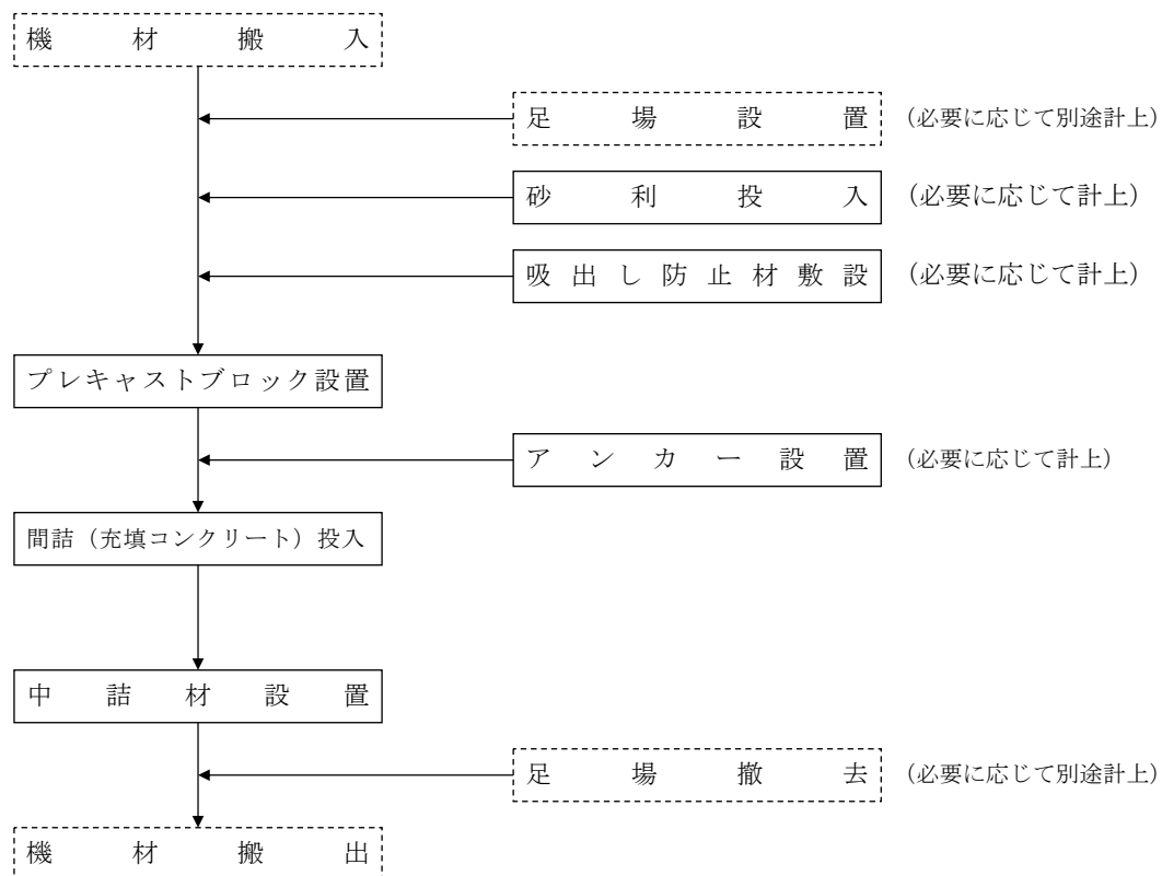
図1－1 施工フロー
