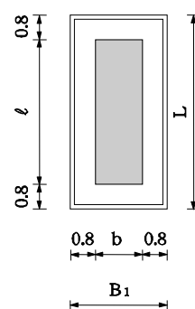
(平面図)
