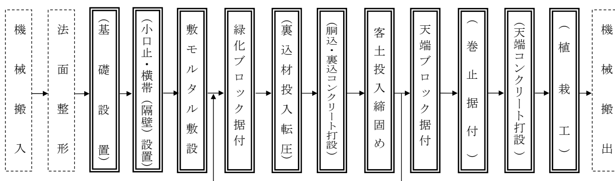
図2-3 施工フロー(緑化ブロック積工)
