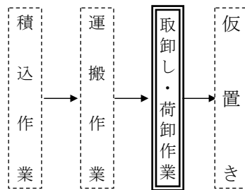
図2－1 施工フロー
