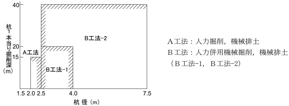
図1－1 適用杭径及び掘削深(標準)
