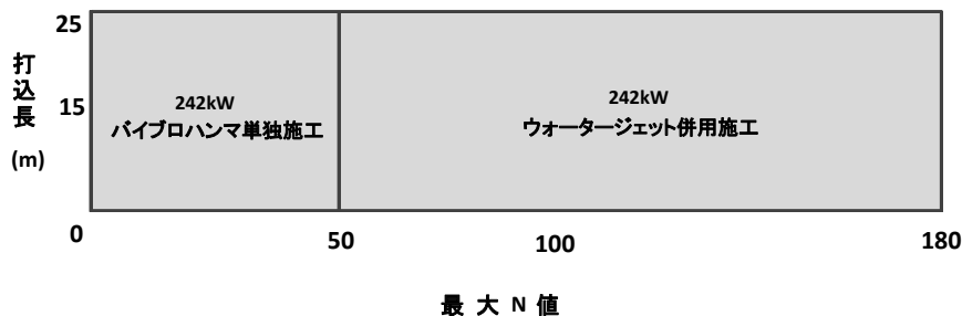
図3-2 油圧式バイブロハンマ 機種を選定範囲
