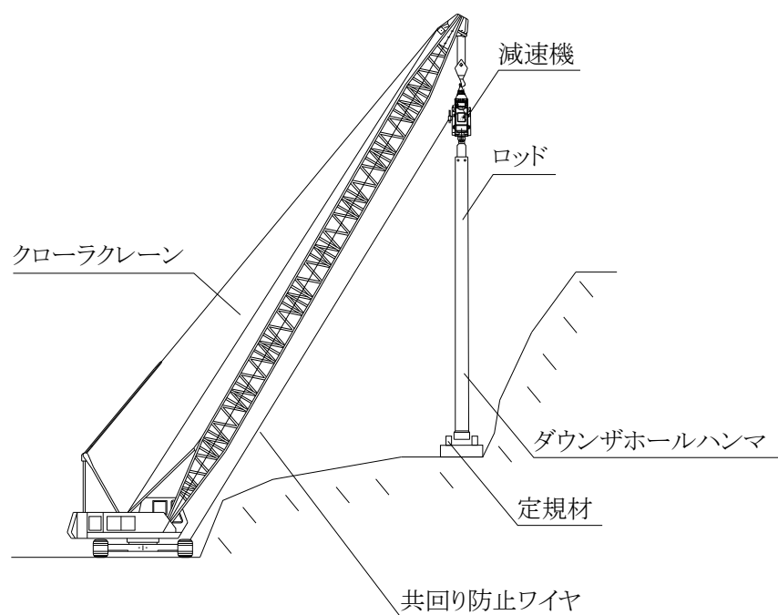
参考図 (A 工法模式図)
