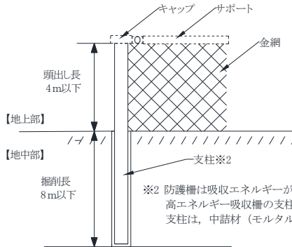
防護柵の場合
