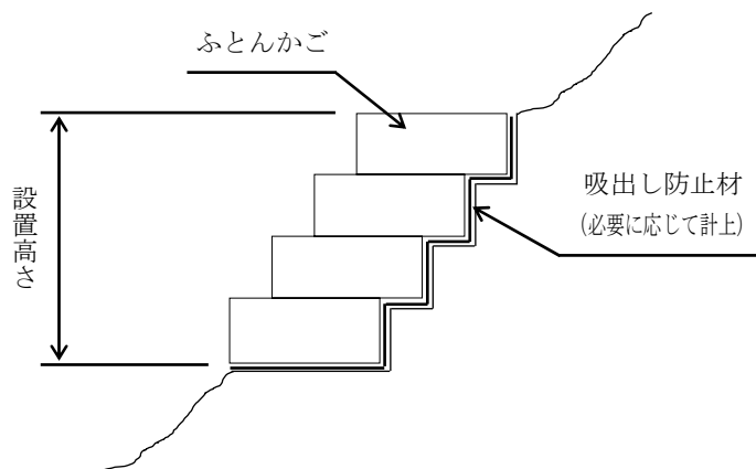
図4-1 地すべり防止工(ふとんかご) 概念図
