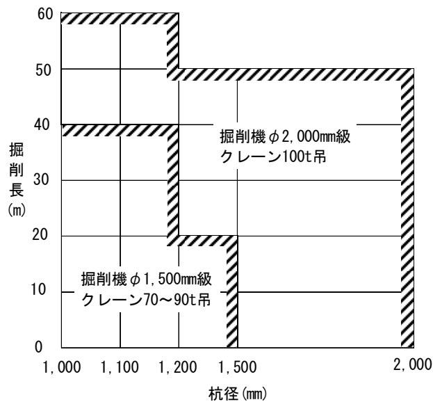
図3-1 全回転型オールケーシング掘削機とクローラークレーンの選定図
