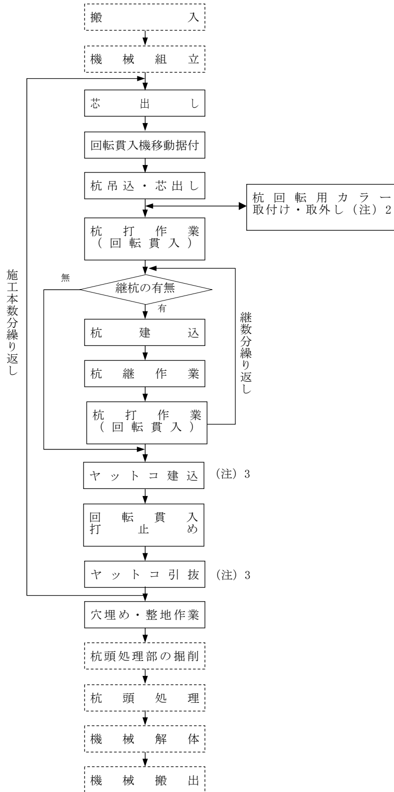
図 2-1 施工フロー
