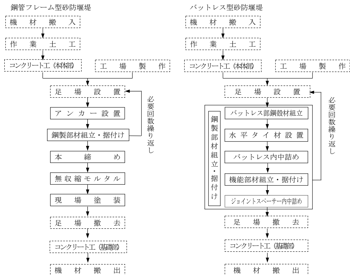
図2-1 施工フロー
