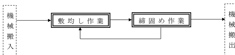
図2-2 施工フロー(路体(築堤)盛土(ICT), 路床盛土(ICT))
