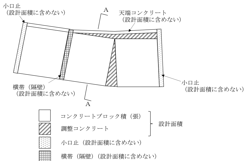
正面図
