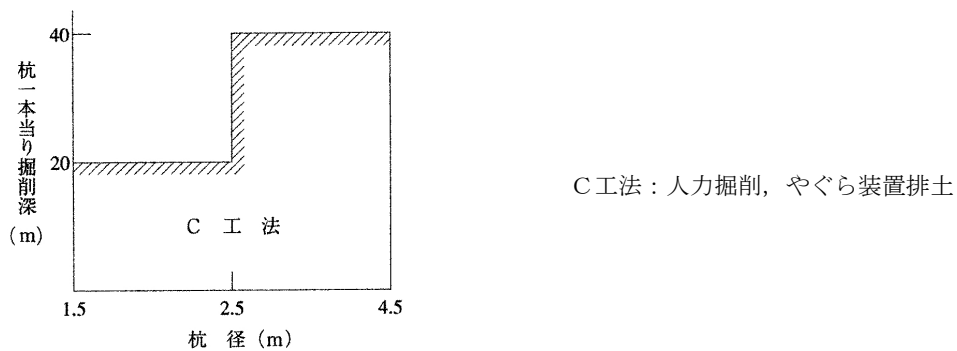
図1－2 適用杭径及び掘削深(掘削機が現場に搬入出来ない場合)
