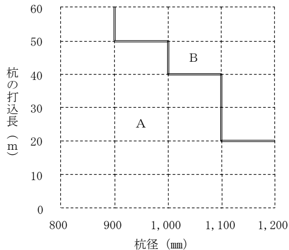
図3-1 クローラ式アースオーガの選定
