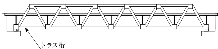
【側面図】
