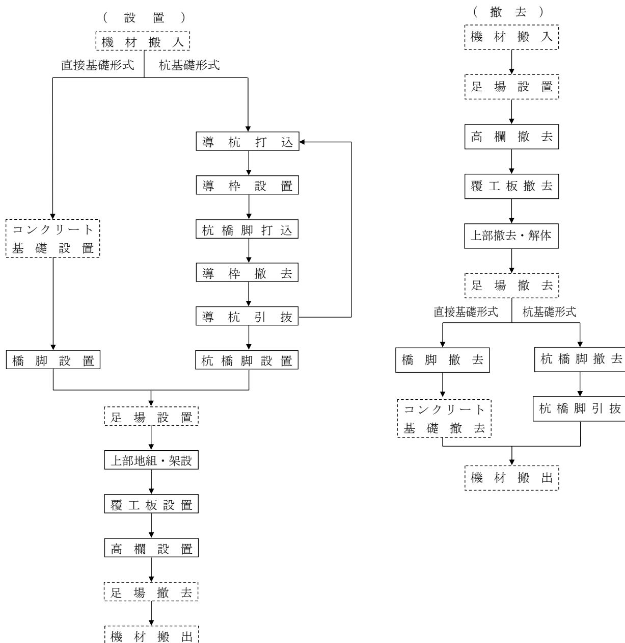
図2-1 施工フロー
