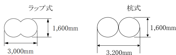
図5-3 改良断面図
