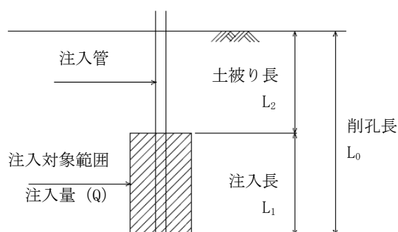
図3-1 施工図
