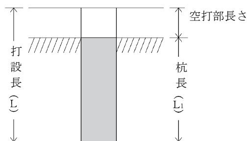
図3-1 施工図
