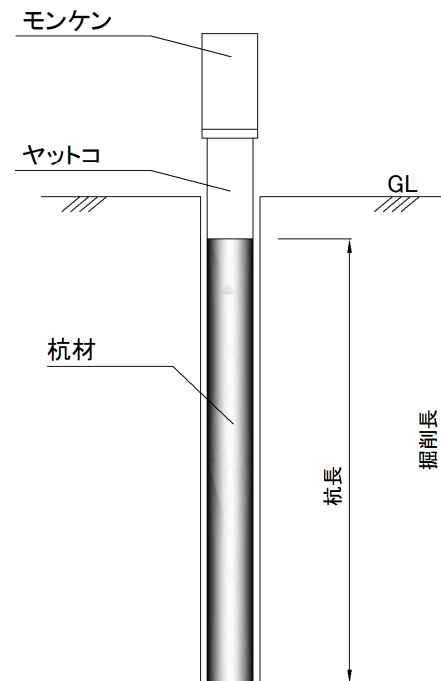
図1-2 施工図(打撃)
