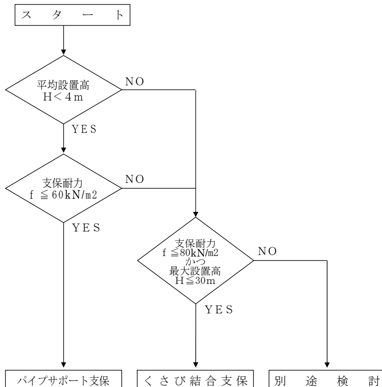
図2－2 工法の選定
