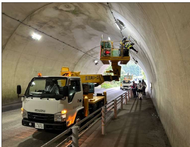
高所作業車による点検状況（内部肩部）
