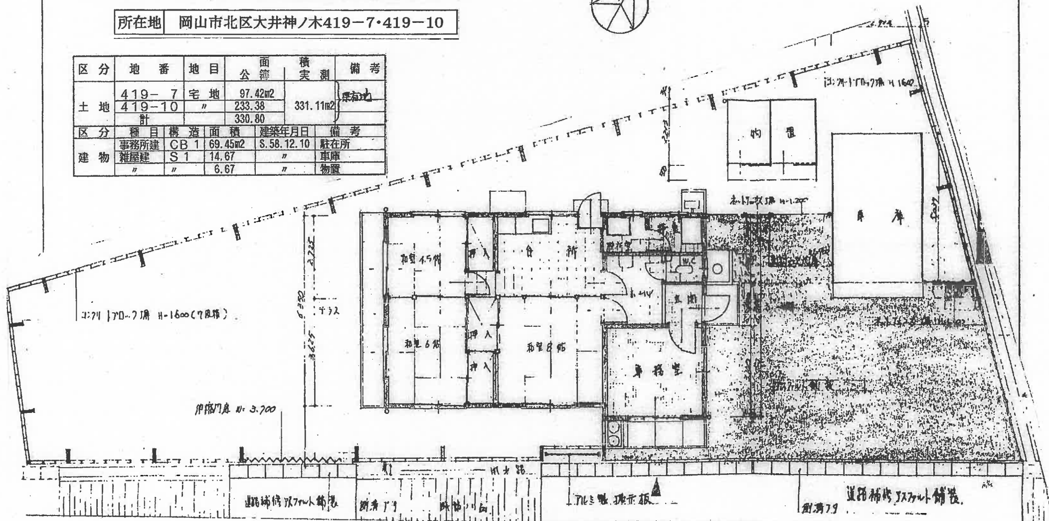
岡山西警察署・大井駐在所配置平面図 S=1:100
