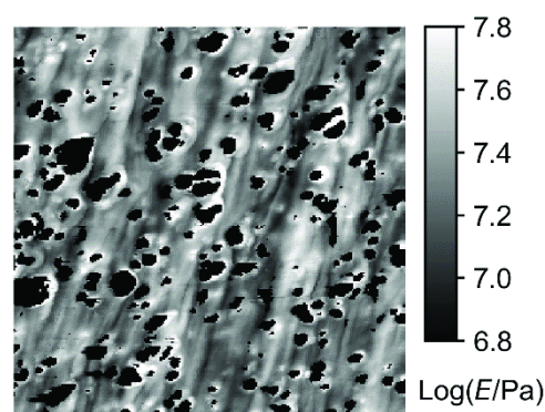
図3 CBを黒色でマスク処理したJKR弾性率像(CB-40の400%伸長)、スキャンサイズは2 \mu\text{m}
