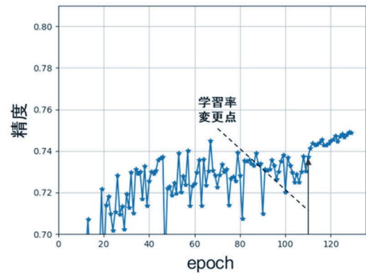
図4 従来学習法による生徒モデルの推定精度
