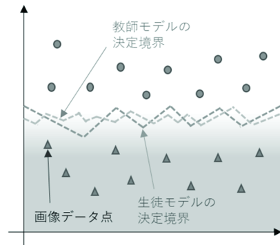
図2 従来蒸留による決定境界のイメージ
