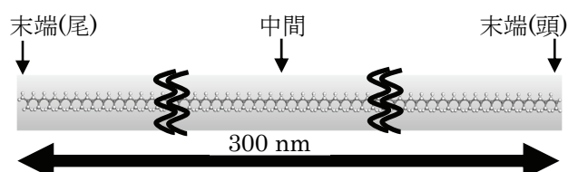
図1 2000量体のPP(アイソタクチック構造)の計算モデル
