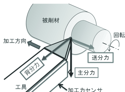
図1 旋削加工の模式図
