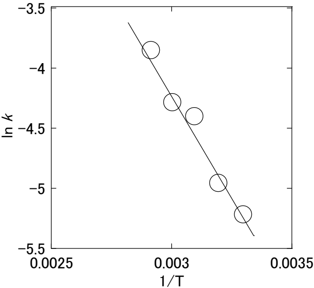
図 3 不溶化反応の温度依存性
