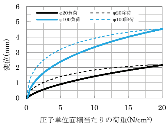
図 5 畳（稲わら畳床）の圧縮曲線
