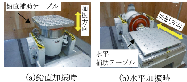
図1 振動試験機
