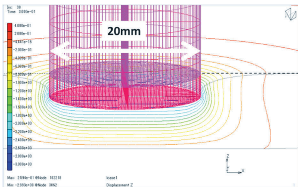
図 4 等方性材料の有限要素解析結果
