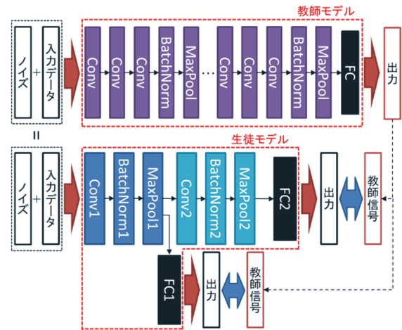
図1 提案蒸留の流れ
