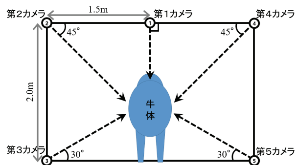
図2 牛体測定システムのカメラ配置
