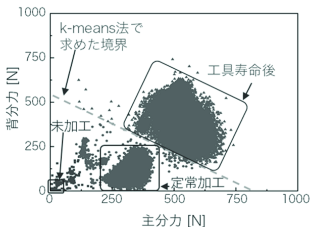
図3 加工力の分布とk-means法から求めた境界線
