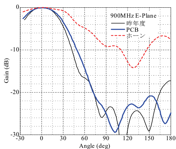
図7 アンテナ指向性
