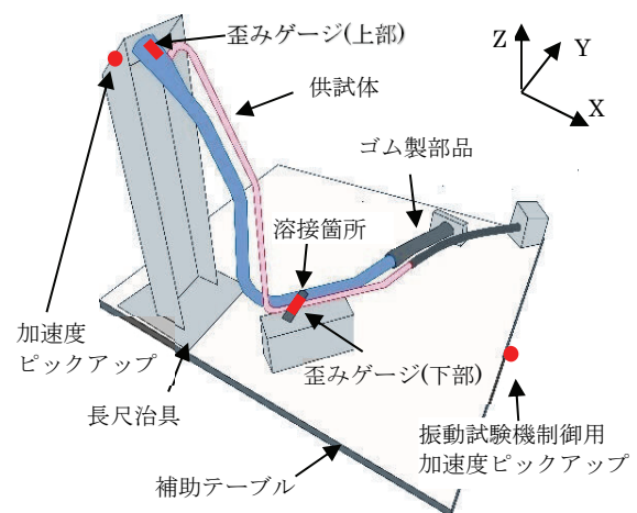
図2 供試体およびセンサの配置図
