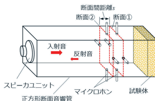
図1 正方形断面音響管による8マイクロホン法垂直入射吸音率測定の概要
