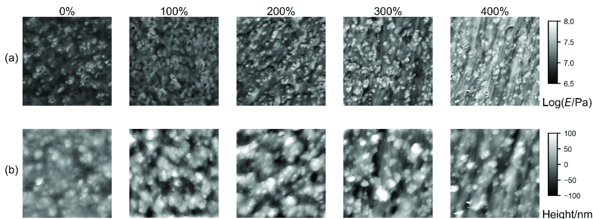
図2 CB-40の各伸長比における (a) JKR弾性率像, (b)高さ像、スキャンサイズは2 \mu\text{m}
