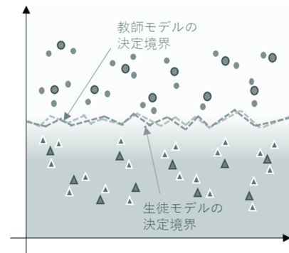
図3 提案蒸留による決定境界のイメージ
