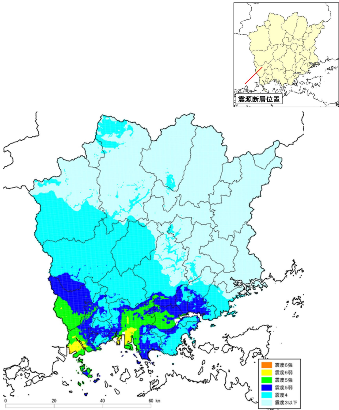
図 6.1.1 震度分布
