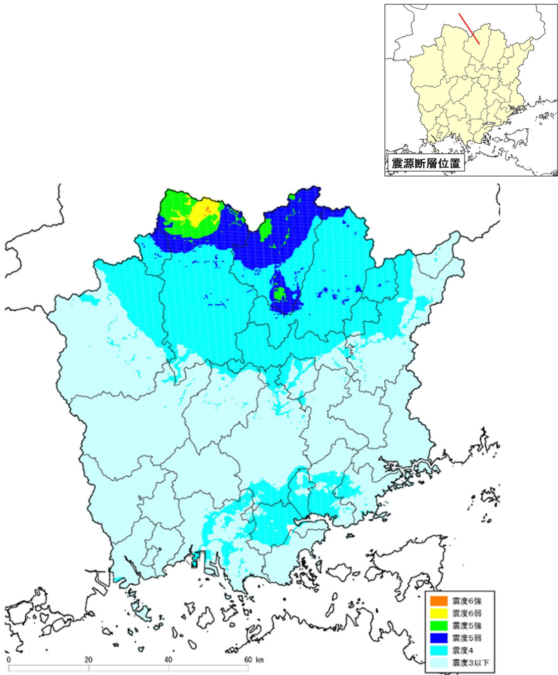
図 8.1.1 震度分布
