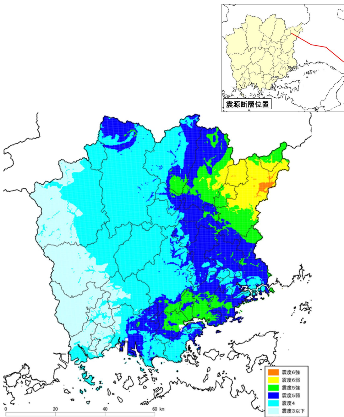
図 3.1.1 震度分布
