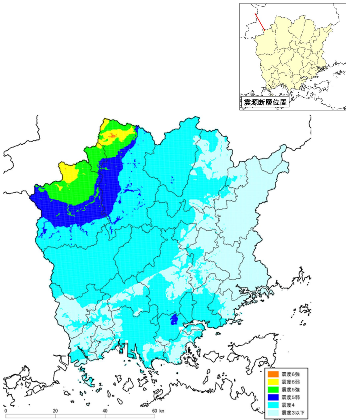
図 9.1.1 震度分布
