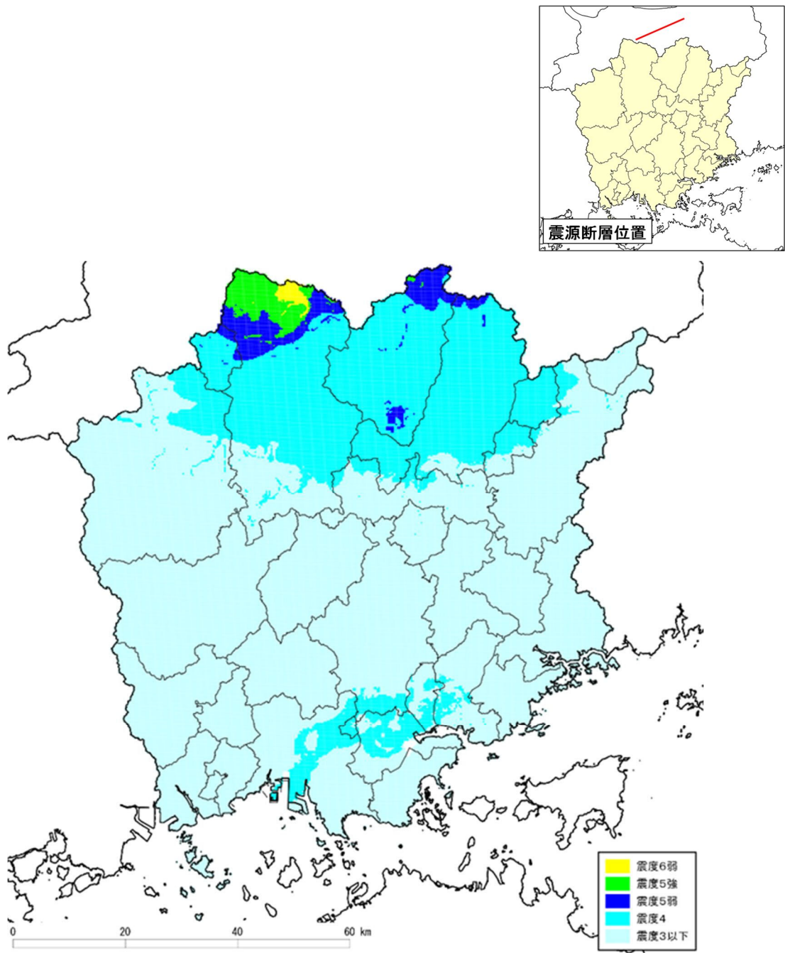
図 7.1.1 震度分布
