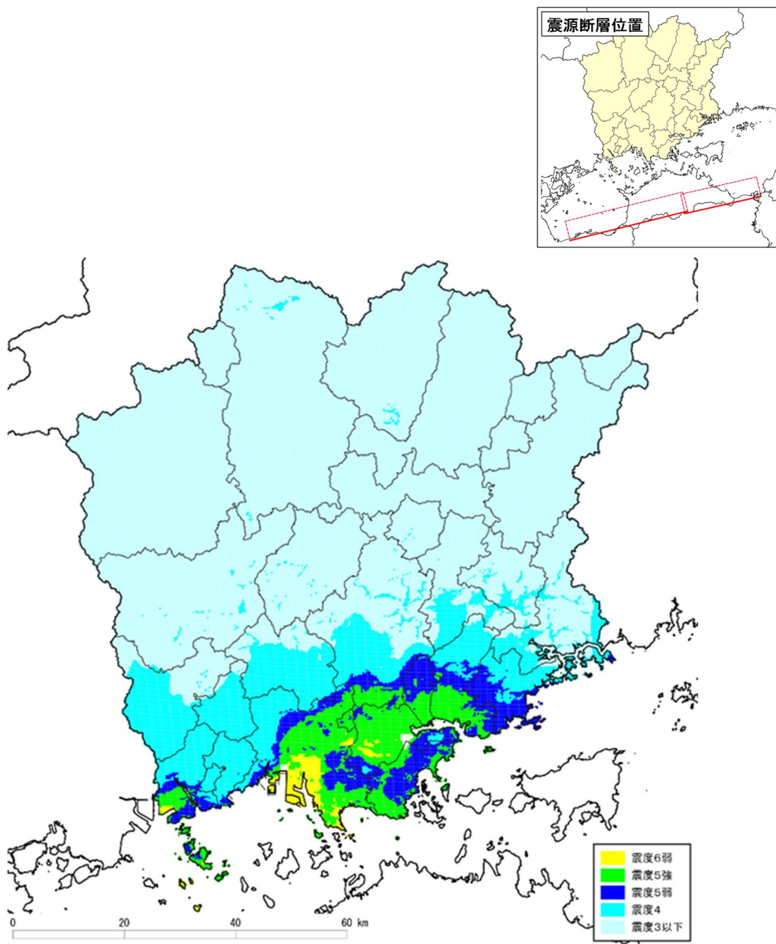
図 5.1.1 震度分布
