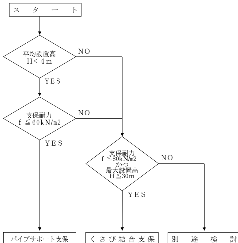
図2－2 工法の選定
