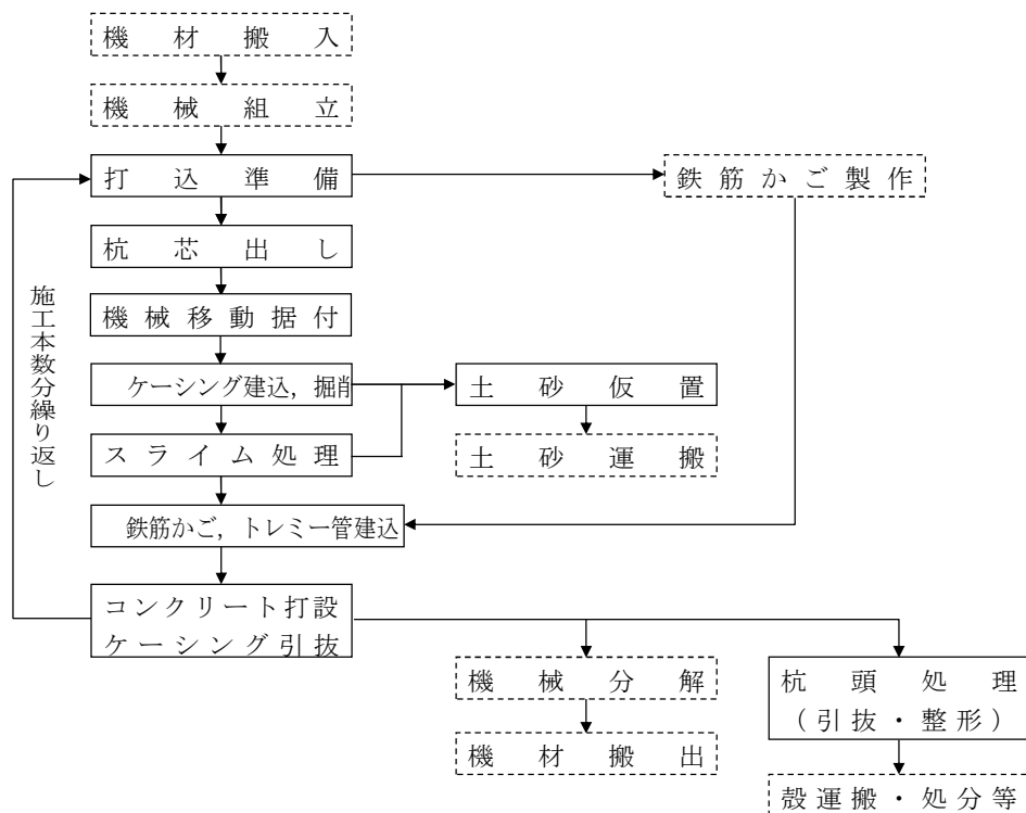
図2－1 施工フロー
