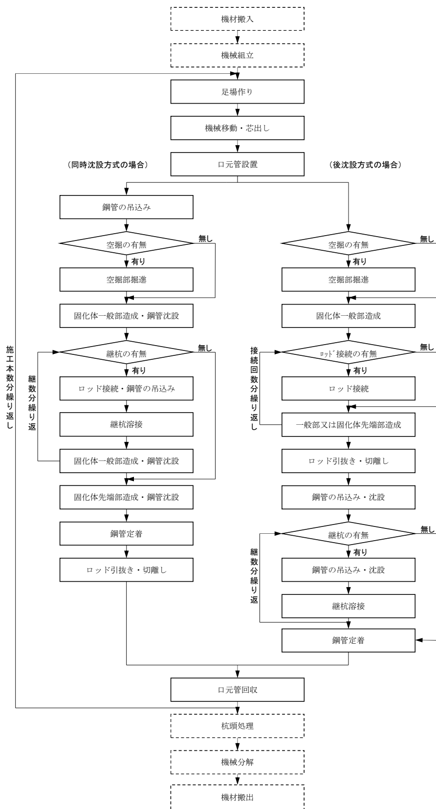
図2-2 施工フロー
