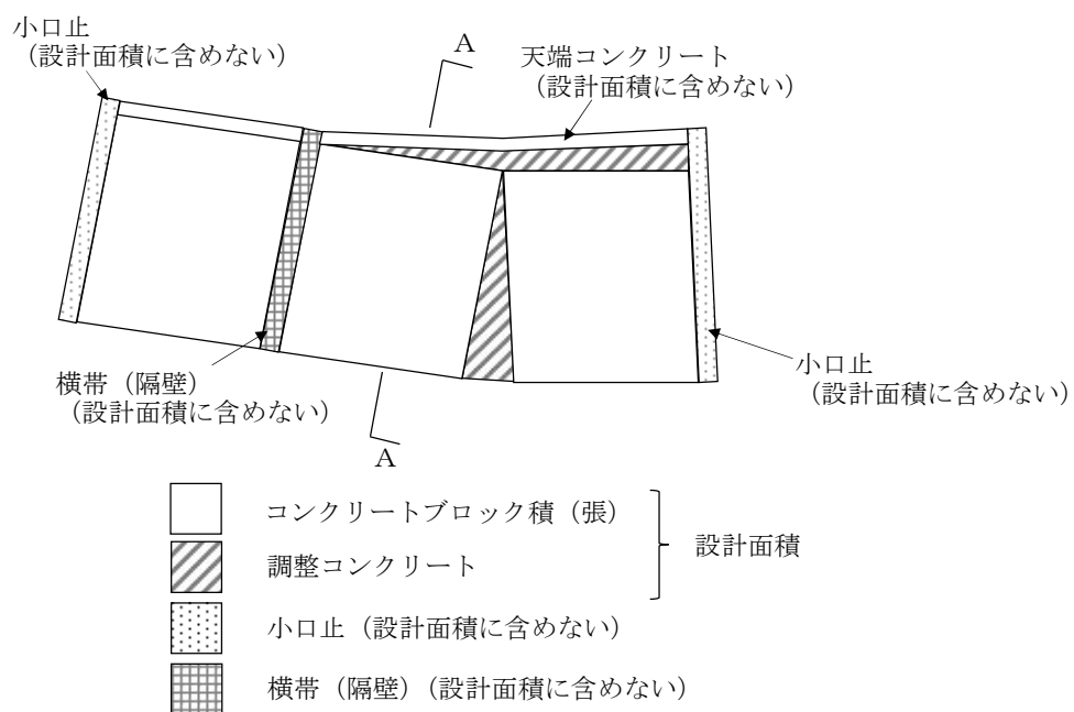
正面図
