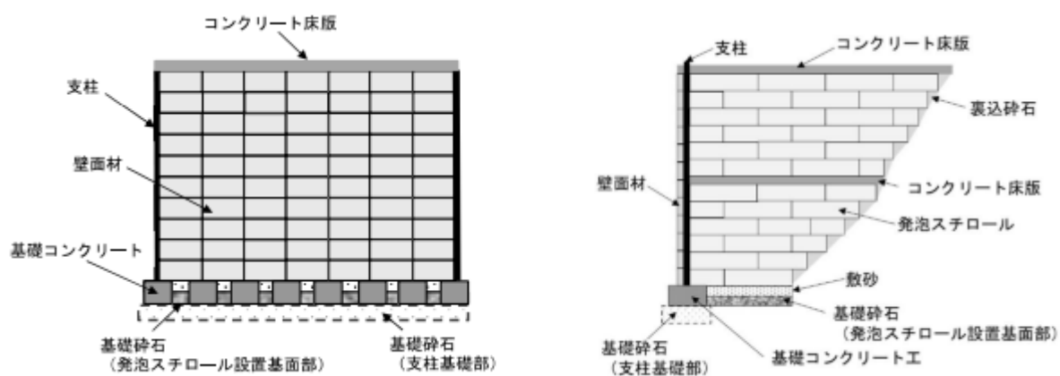
片側壁図
