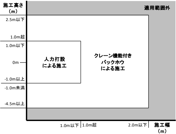
図2－3 コンクリート打設工法の選定(防草コンクリート)
