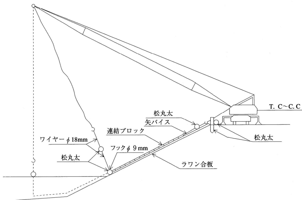
図5-2 連節ブロック水中吊落し断面図
