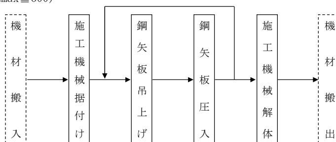
図2-2 施工フロー(圧入( N_{max} \leq 50 ))
