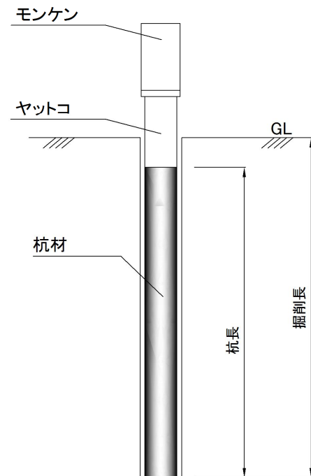
図1-2 施工図(打撃)
