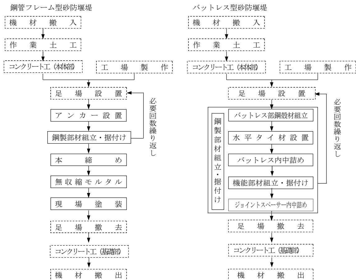
図2-1 施工フロー
