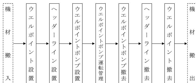
図2-1 施工フロー
