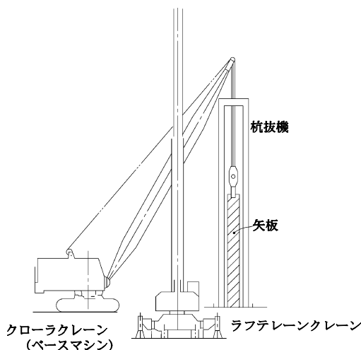
図2-2 施工図
