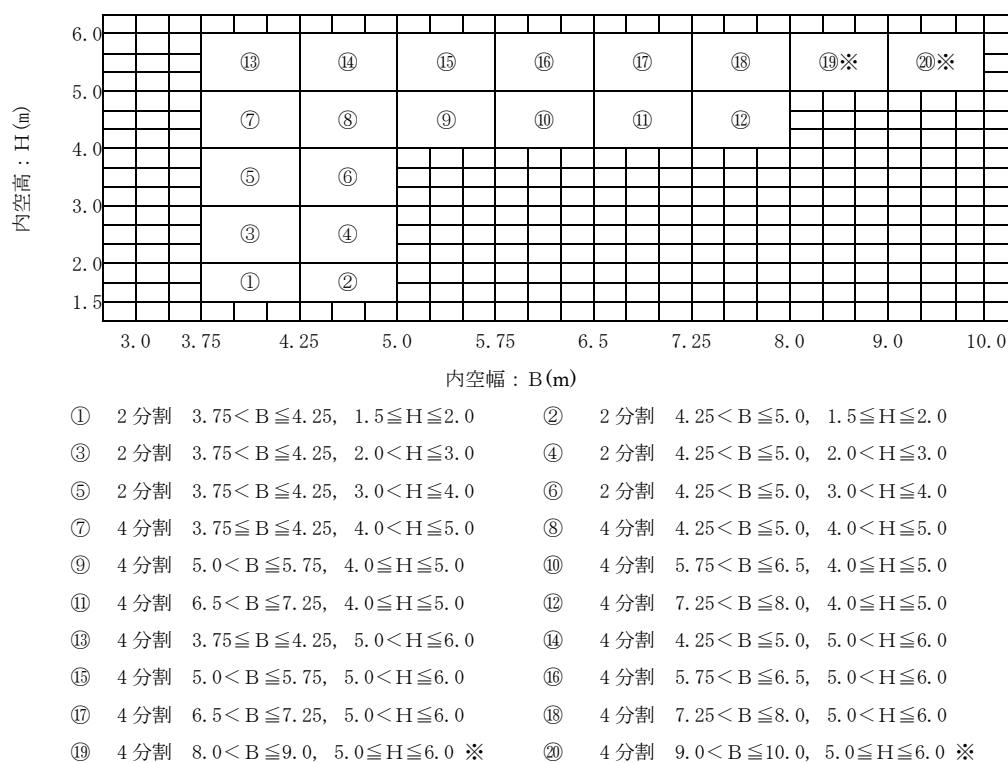
図4-1 大型プレキャストボックスカルバートの歩掛区分
