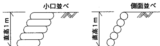
図2-1 施工図
