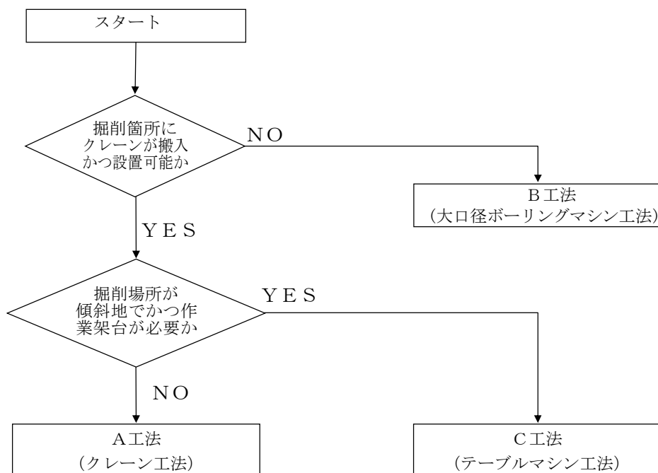
図2-4 工法の選定
