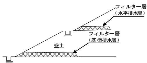
フィルター層の参考図
