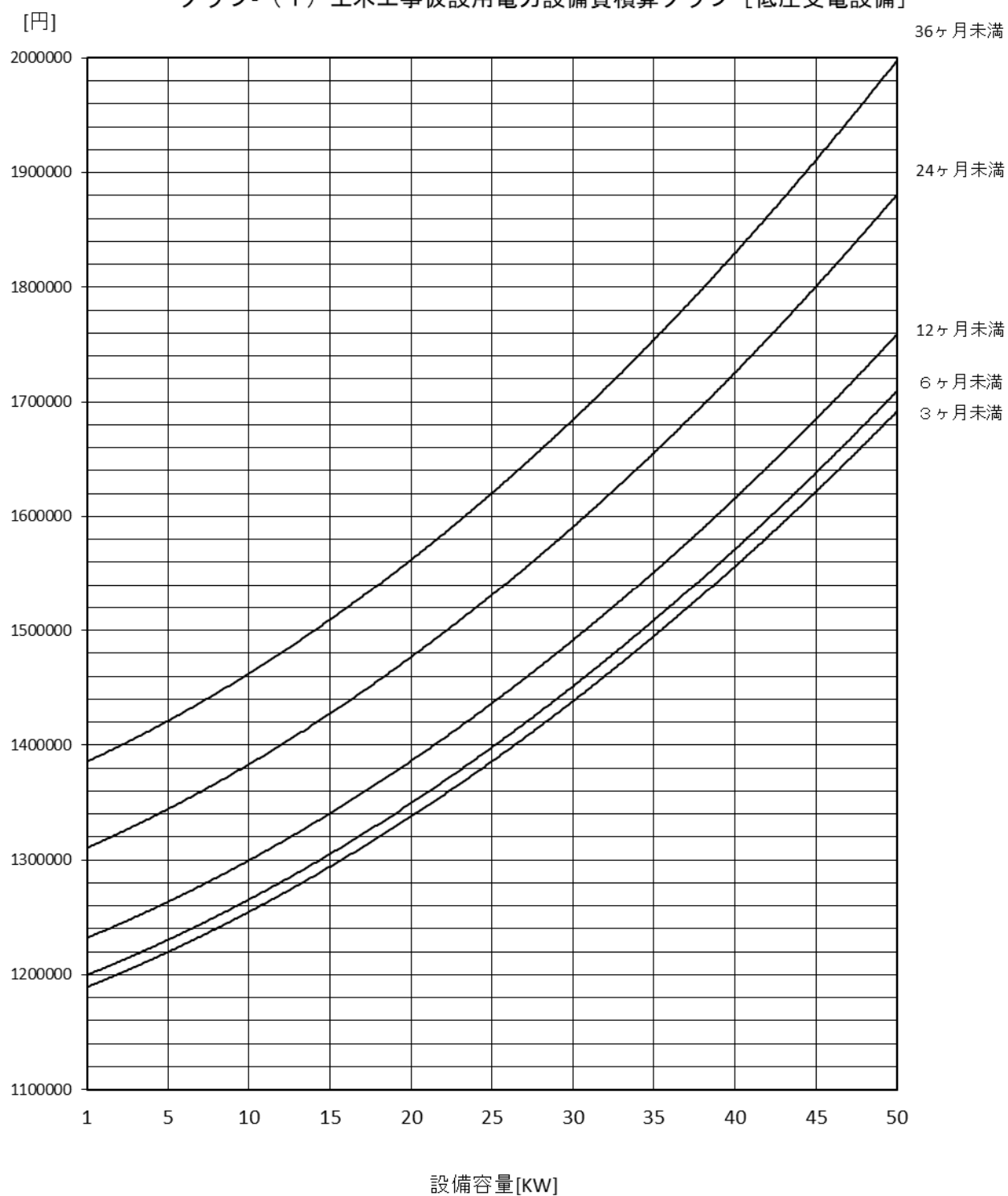
グラフ-（１）土木工事仮設用電力設備費積算グラフ〔低圧受電設備〕
