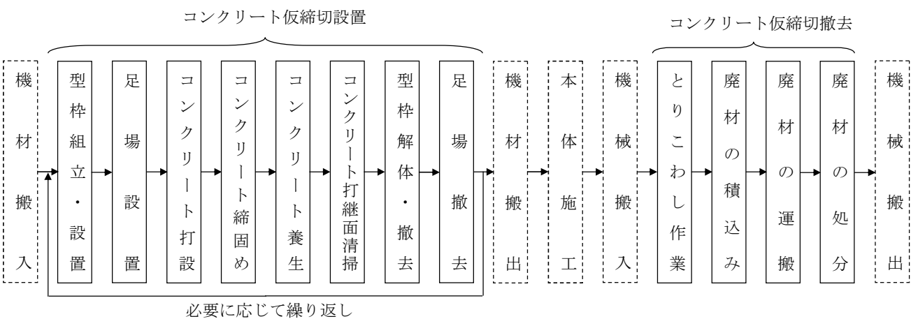
図2－1 施工フロー
