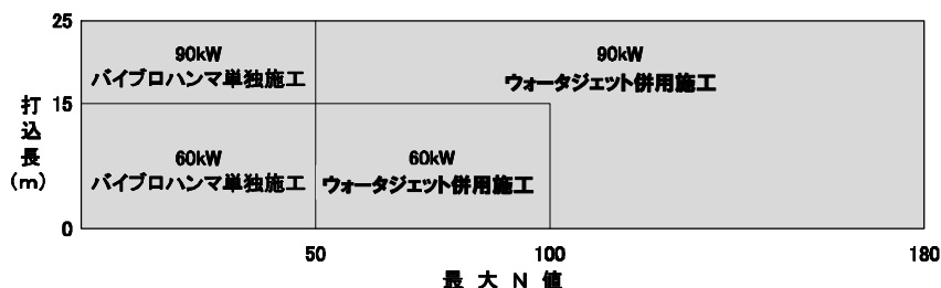
図3-1 電動式バイブロハンマ 機種種の選定範囲
