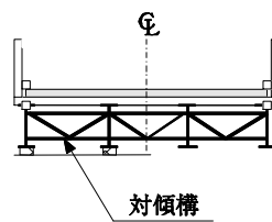
【断面図】
