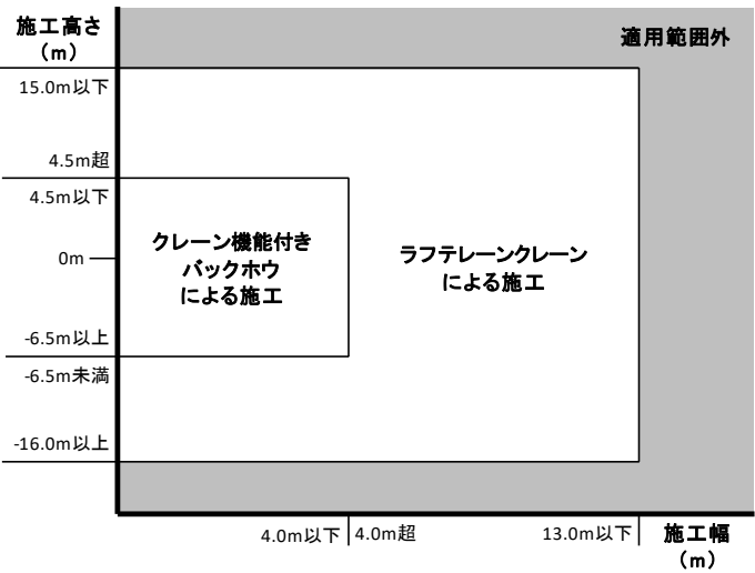
図2－2 コンクリート打設工法の選定(縦排水溝・小段排水溝)
