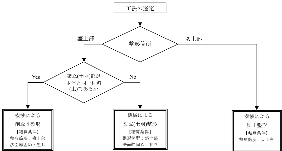
図3－１ 法面整形工(ICT) 工法選定フロー図
