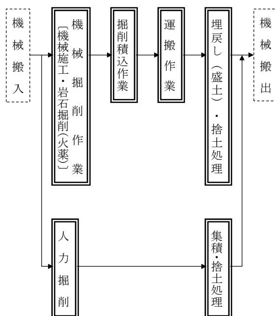
図2-1 施工フロー
