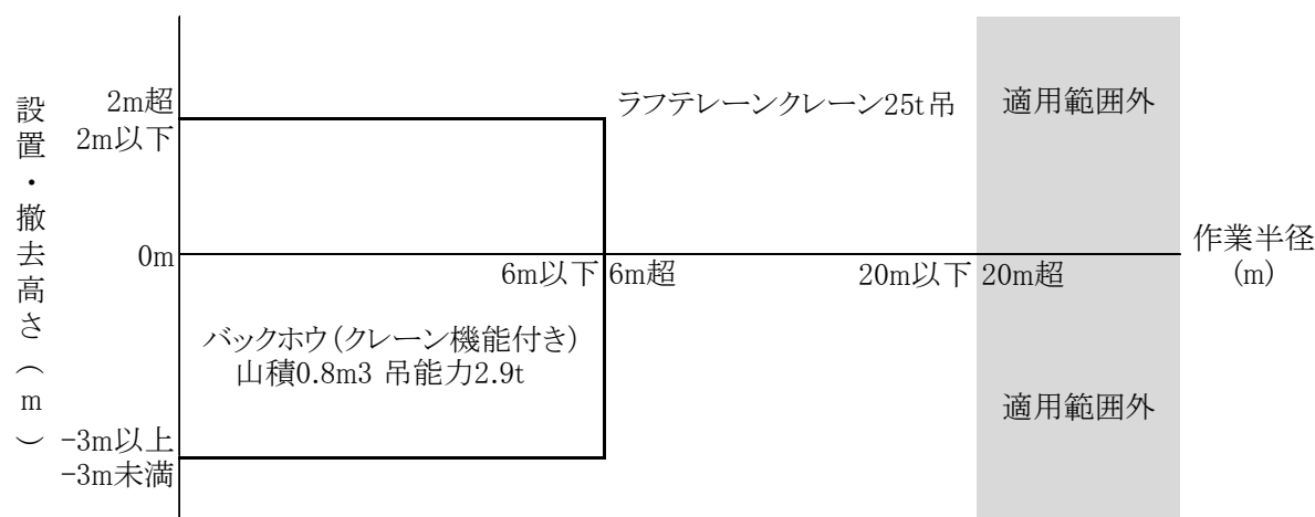
図3-1 機種の選定 製作・設置
