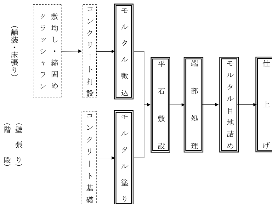
図2-1 施工フロー
