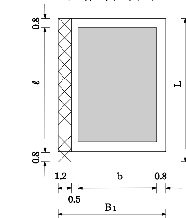
(断面図)
