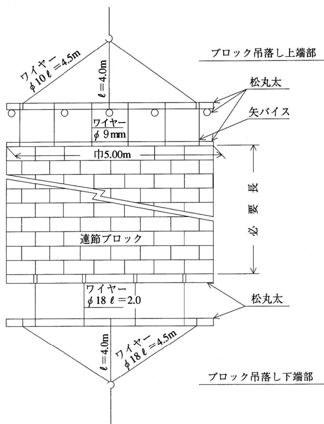
図5-1 連節ブロック水中吊落し平面図
