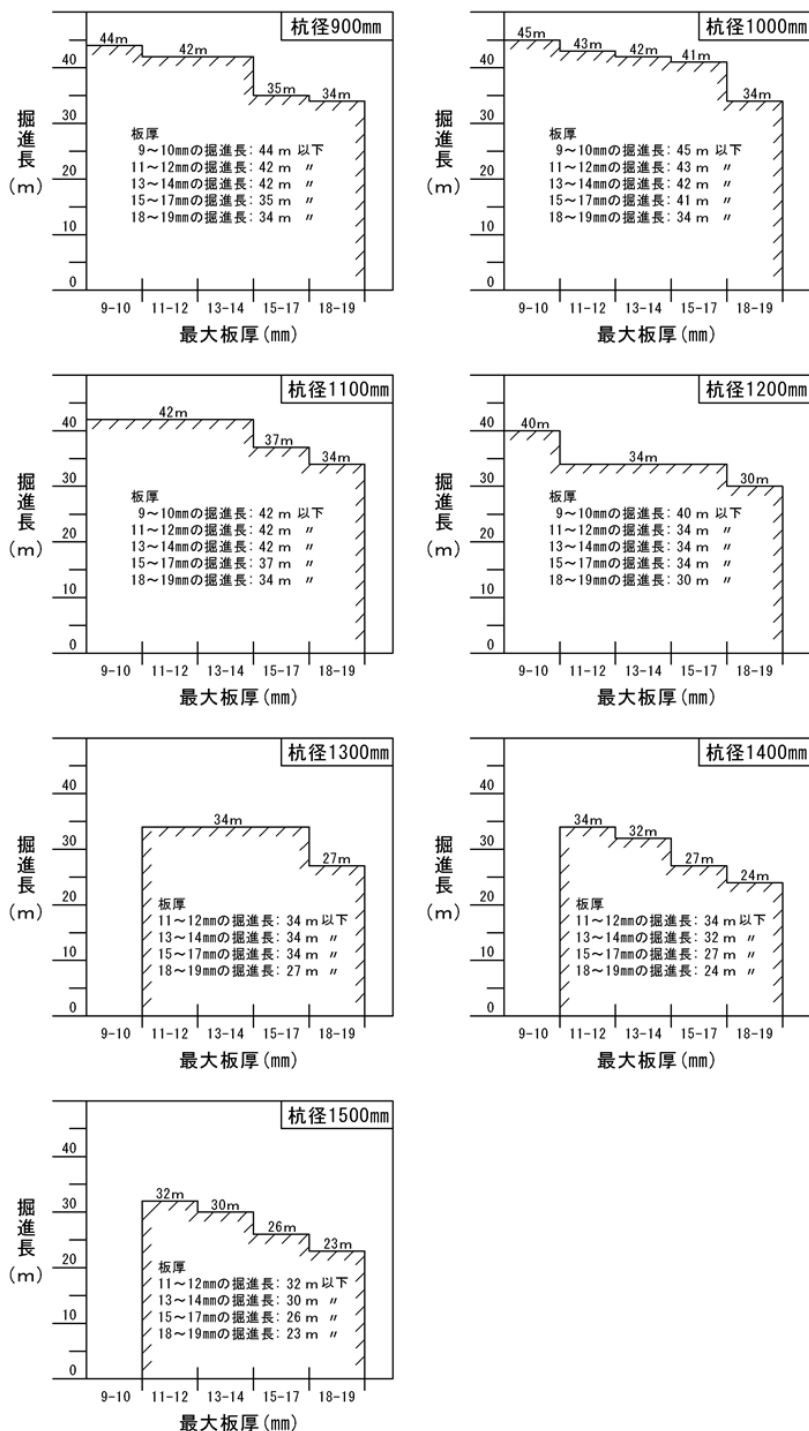
図1ー1 適用掘進長
