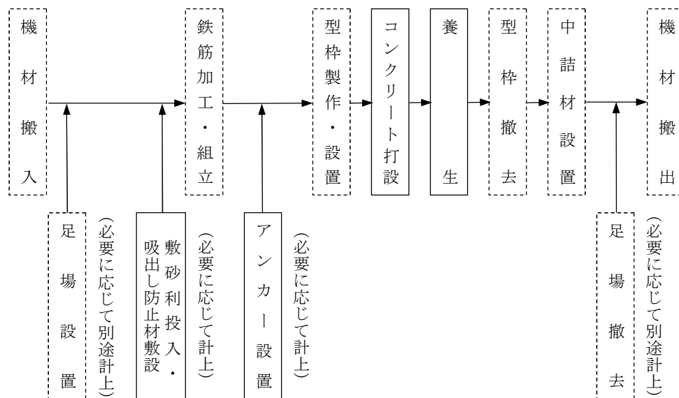
図2－1 施工フロー
