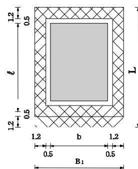
(平面図)
