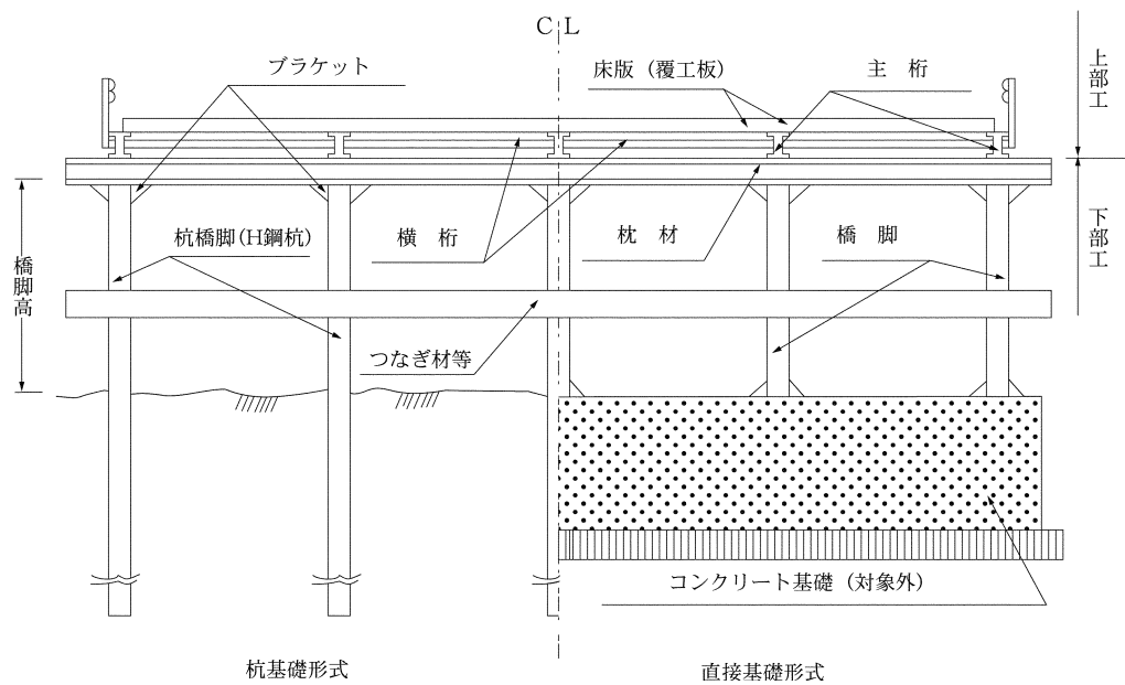
図2-2 仮橋・仮杭橋工概念図
