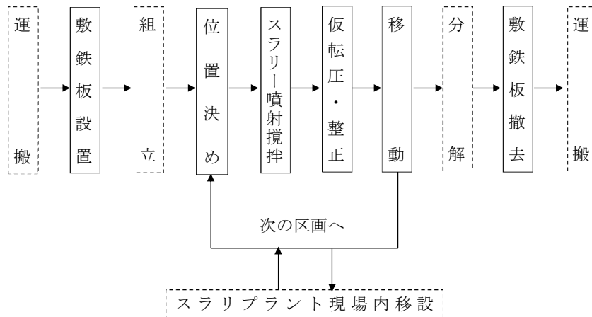
図2-1 施工フロー
