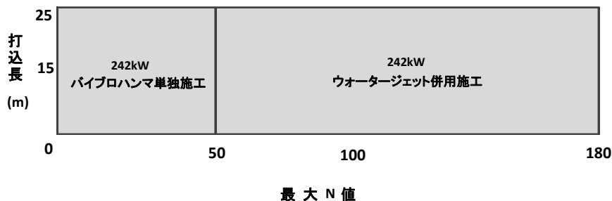
図3-2 油圧式バイブロハンマ 機種種の選定範囲
