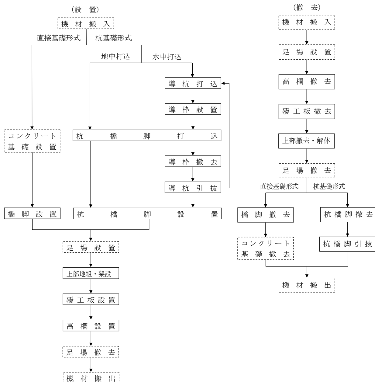
図2-1 施工フロー
