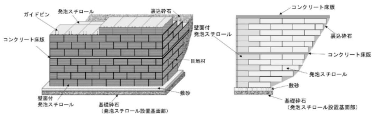
片側壁図
