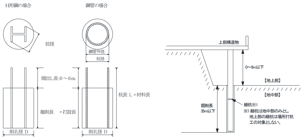
図1-1 施工図
