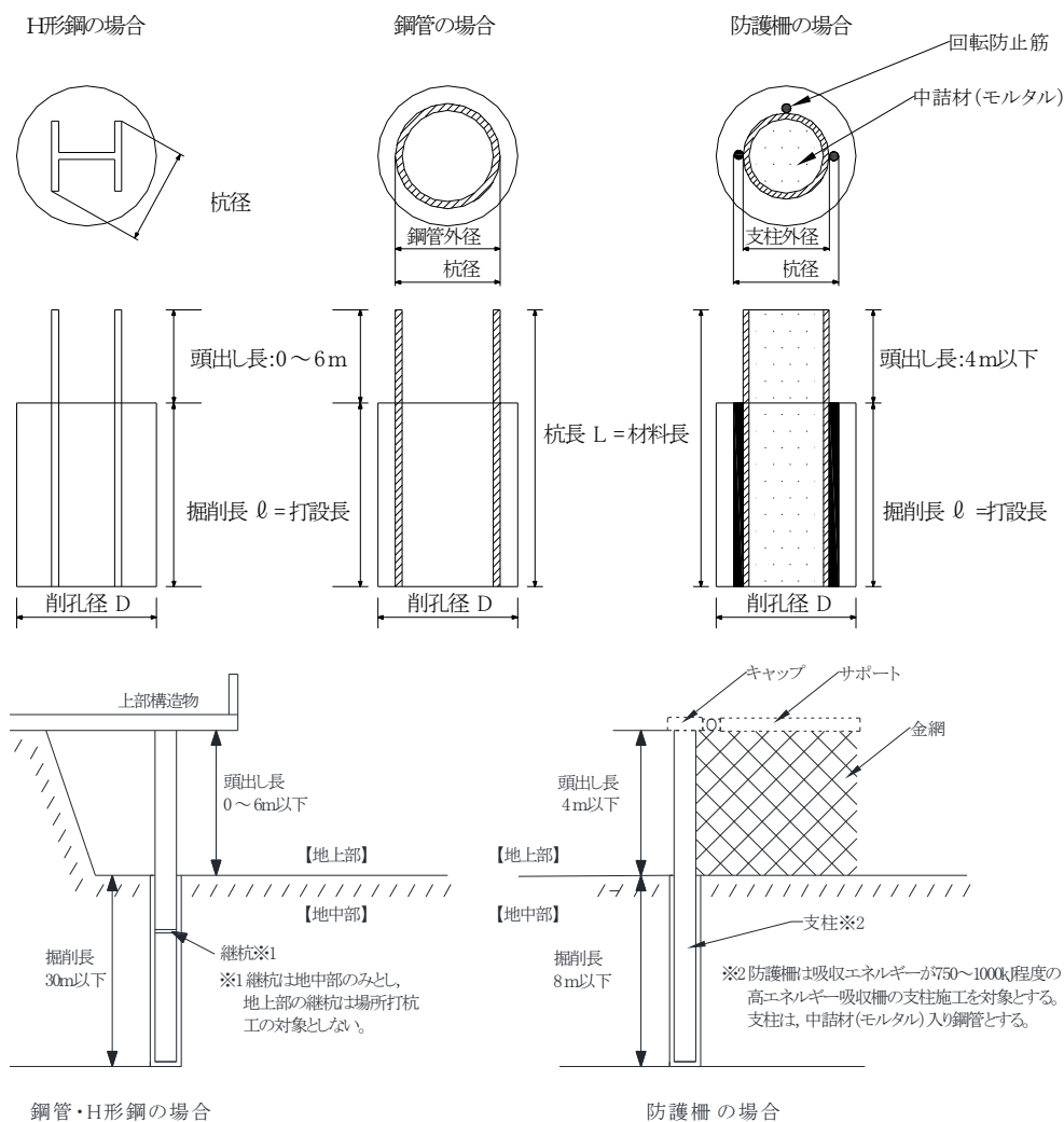
図1-1 施工図
