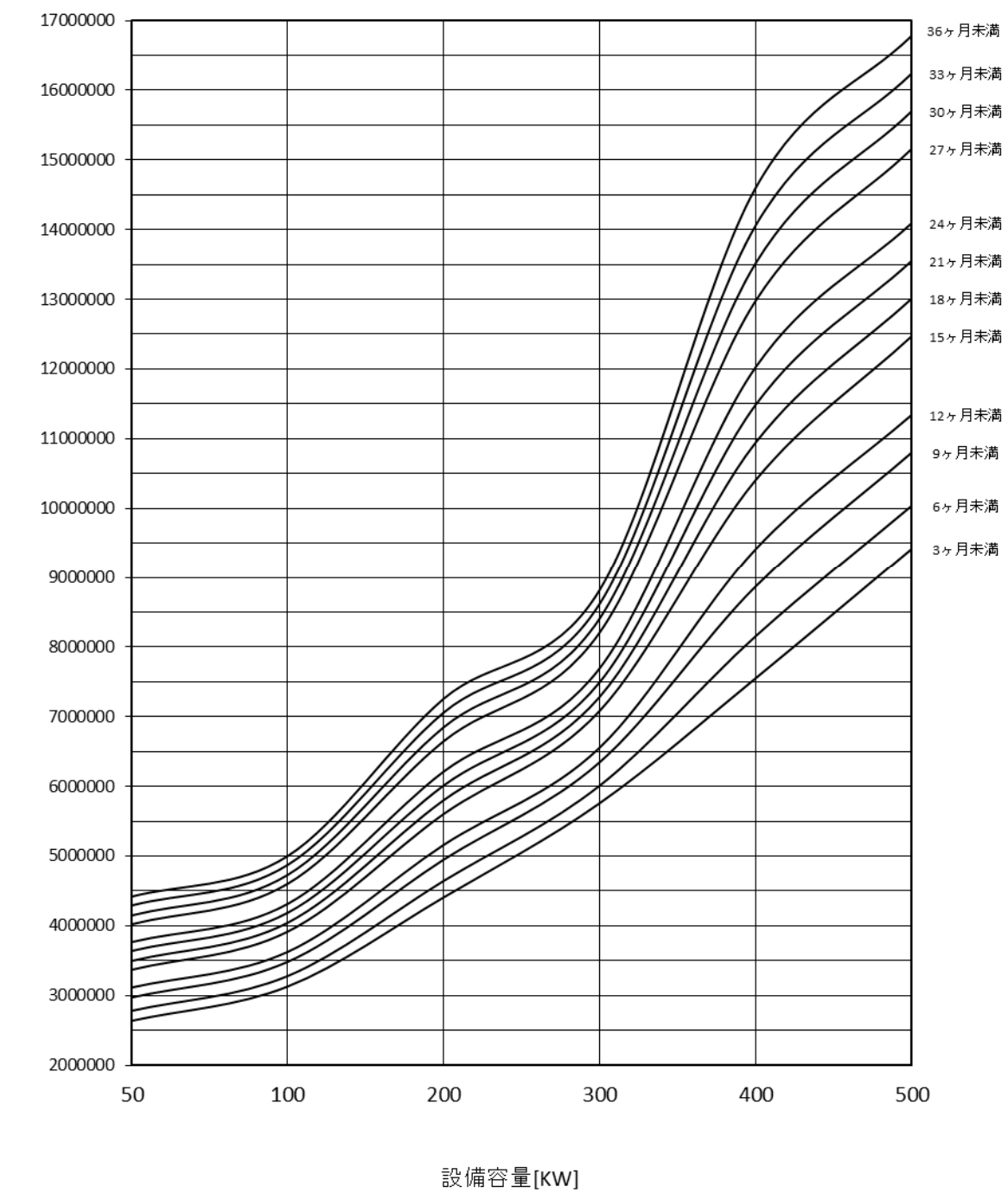
グラフ(2) 土木工事仮設用電力設備費積算グラフ[高压受電設備]
