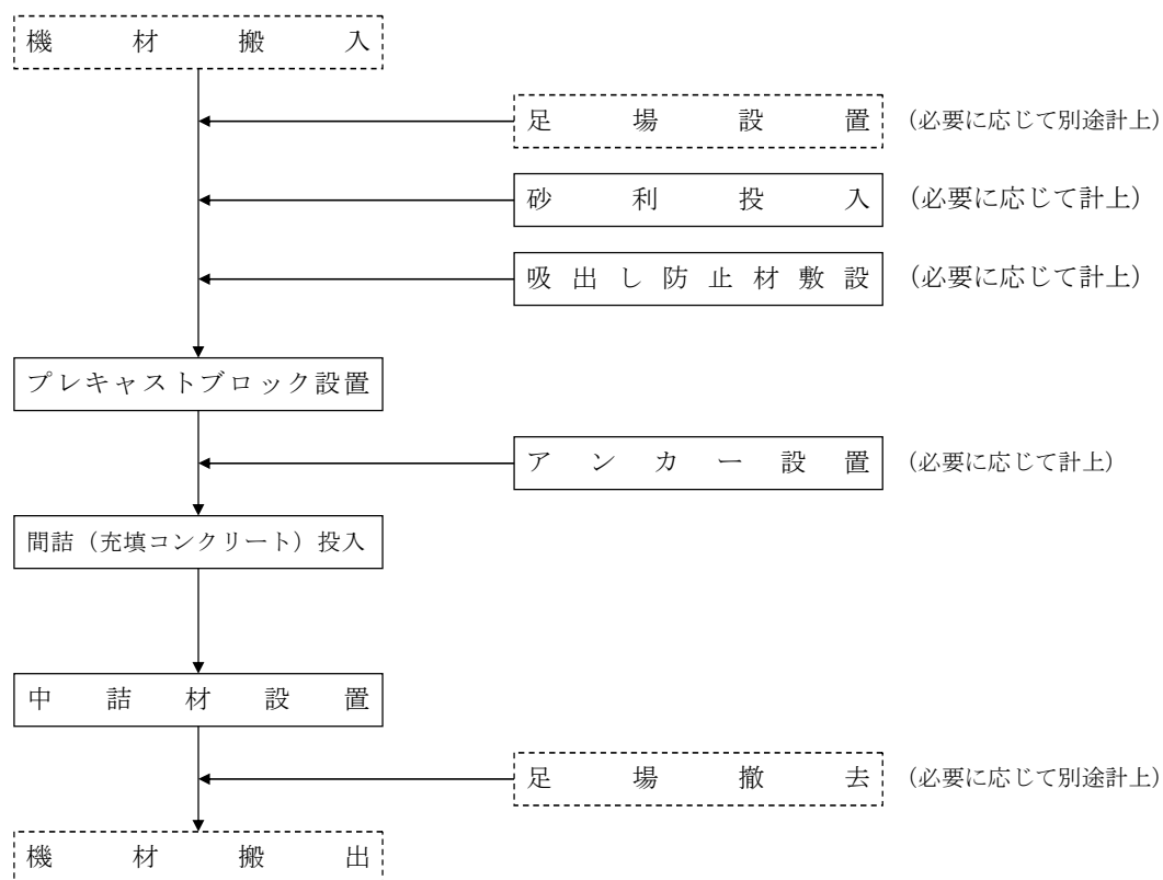
図1－1 施工フロー
