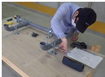
床排水配管実習
