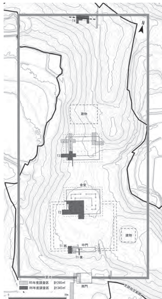
備中国分尼寺跡調査区配置図（1/2,000）
