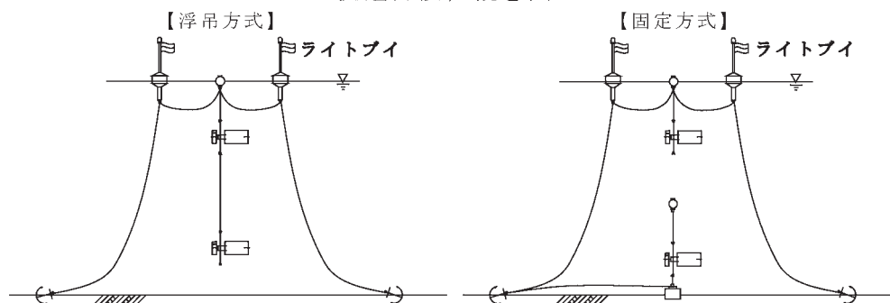
流速計設置概念図
