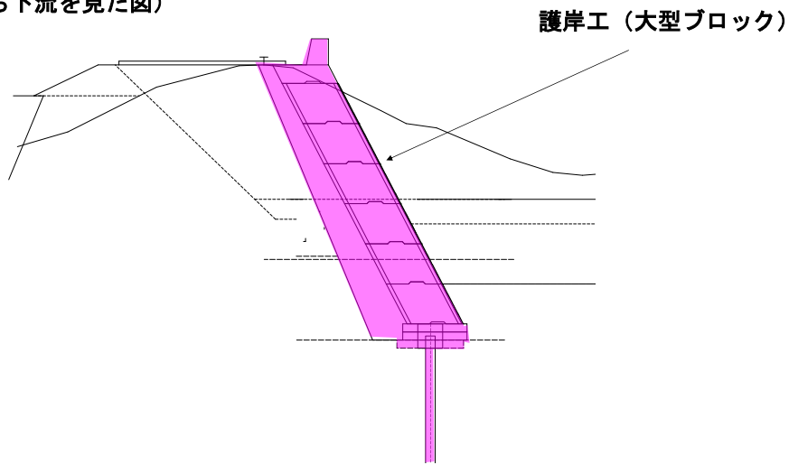
【標準断面図】 （上流から下流を見た図）
