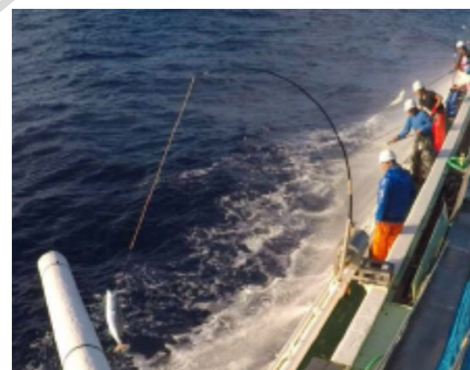
自動かつお釣り機 (かつお一本釣り漁船)
