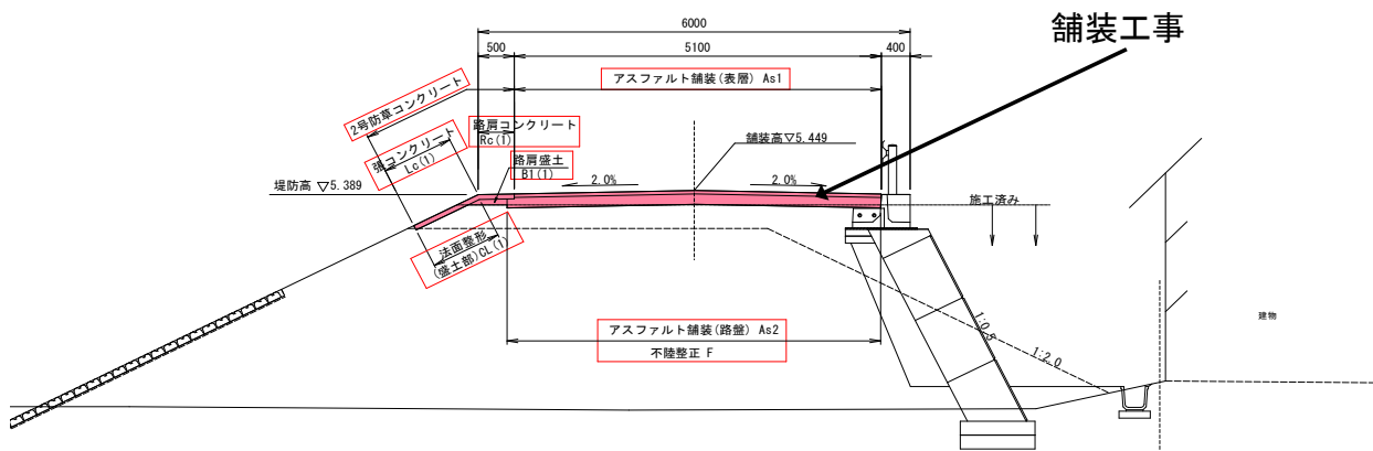
【標準断面図】 (上流から下流を見た図)
