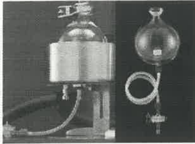
受フラスコ用冷却バス ドレンコック付受フラスコ
