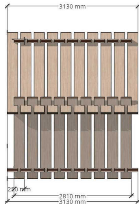
側面図
