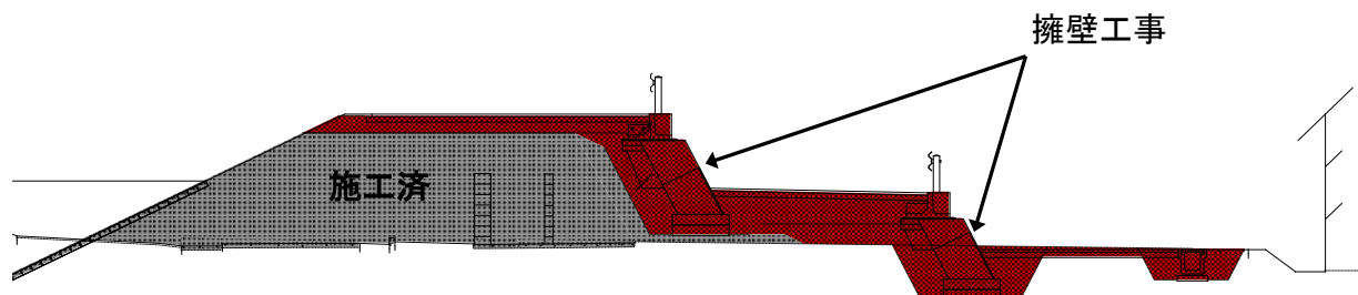
【標準断面図】 (上流から下流を見た図)
