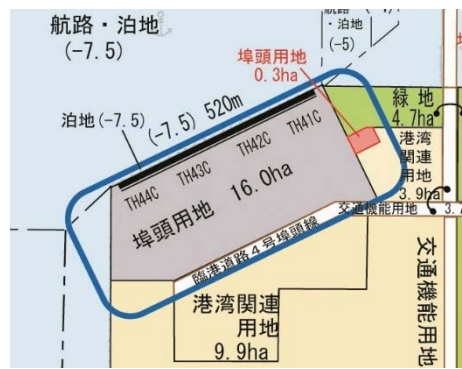
図2-1-1 公共埠頭計画（玉島地区）
