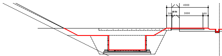
工事横断図
