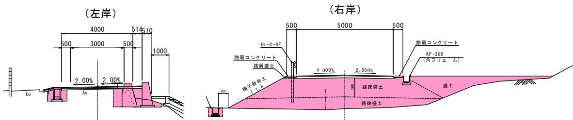
【 工事断面図 】
