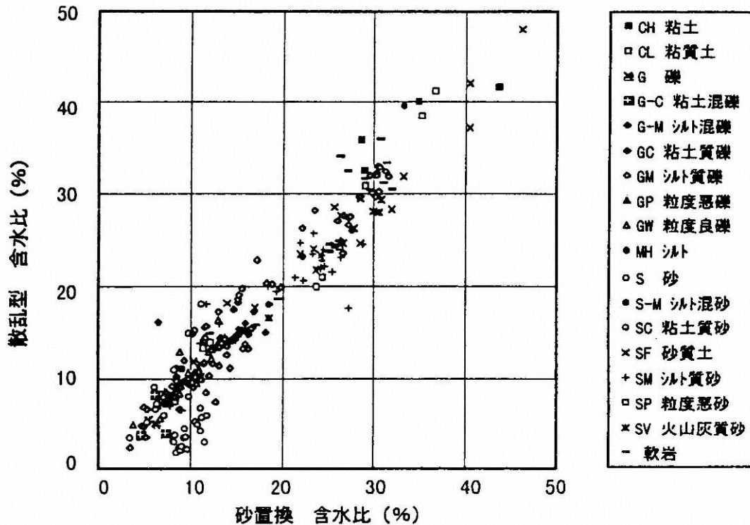
図一 4 砂置換と散乱型の相関 (含水比・土質別データ)
