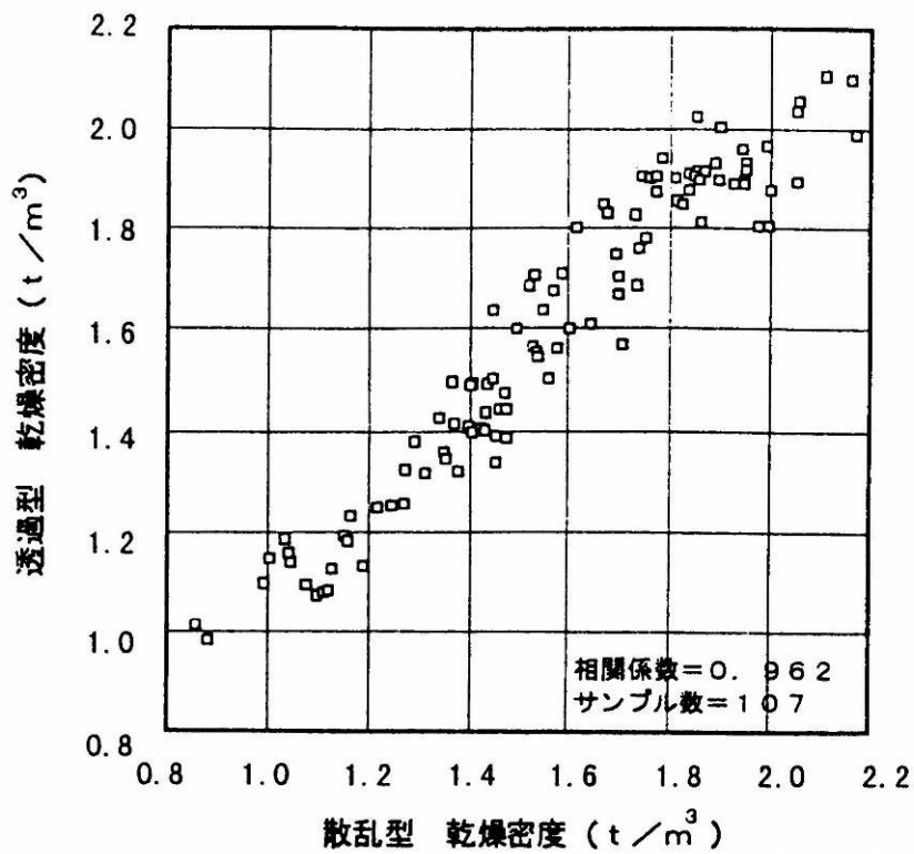
図一9 散乱型と透過型の相関 (乾燥密度・全データ)
