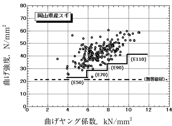
図2 スギ材の曲げ強度と機械等級区分
