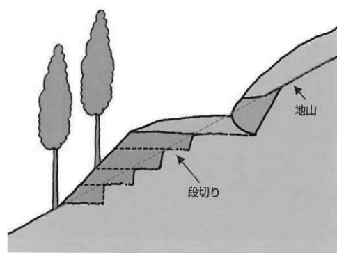
段切段盛のイメージ
