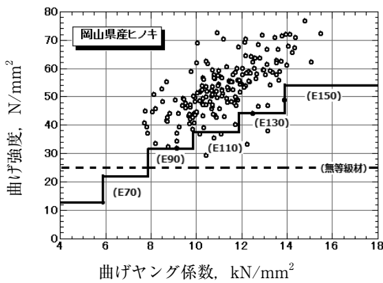
図1 ヒノキ材の曲げ強度と機械等級区分
