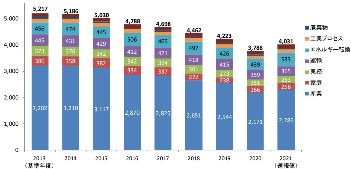
参考1 温室効果ガス排出量の年度推移（単位：万 t-CO 2 ）
