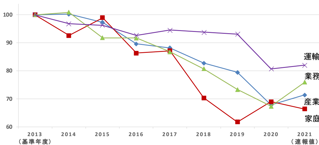
参考2 主要4部門の二酸化炭素排出量の年度推移（平成25(2013)年度を100とする）
