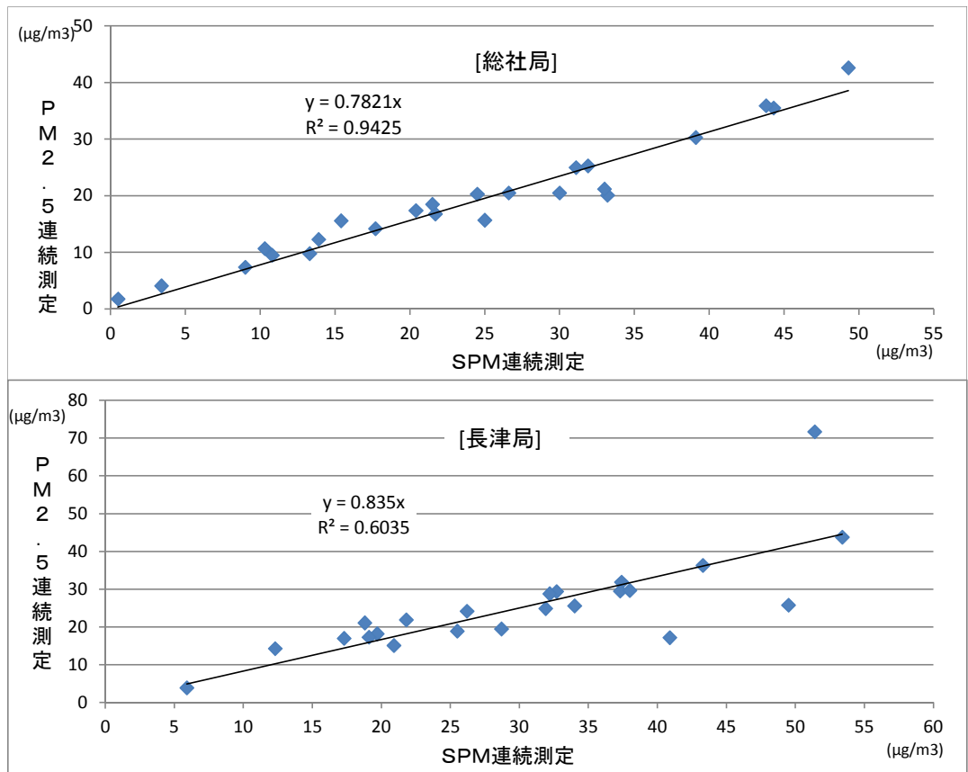
図2 PM2.5連続測定－SPM連続測定の測定値比較
