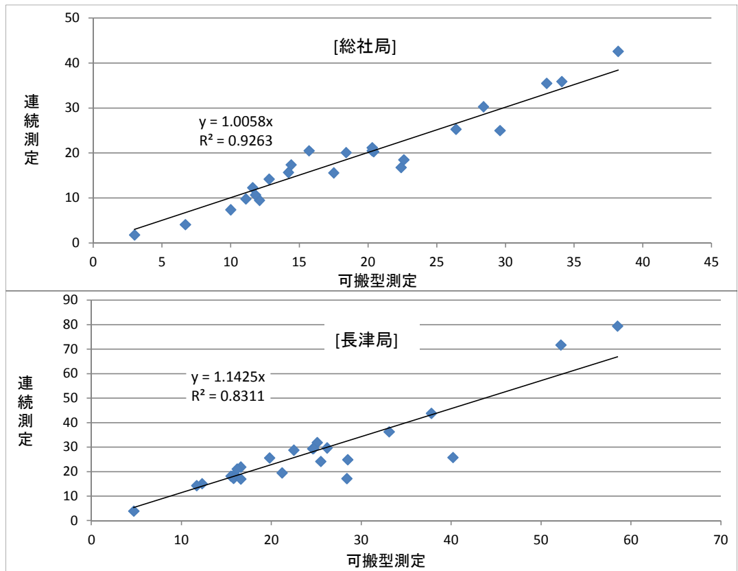
図1 PM2.5可搬型と連続測定の測定値比較
