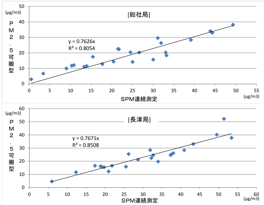
図3 PM 2.5 可搬型—SPM連続測定の測定値比較
